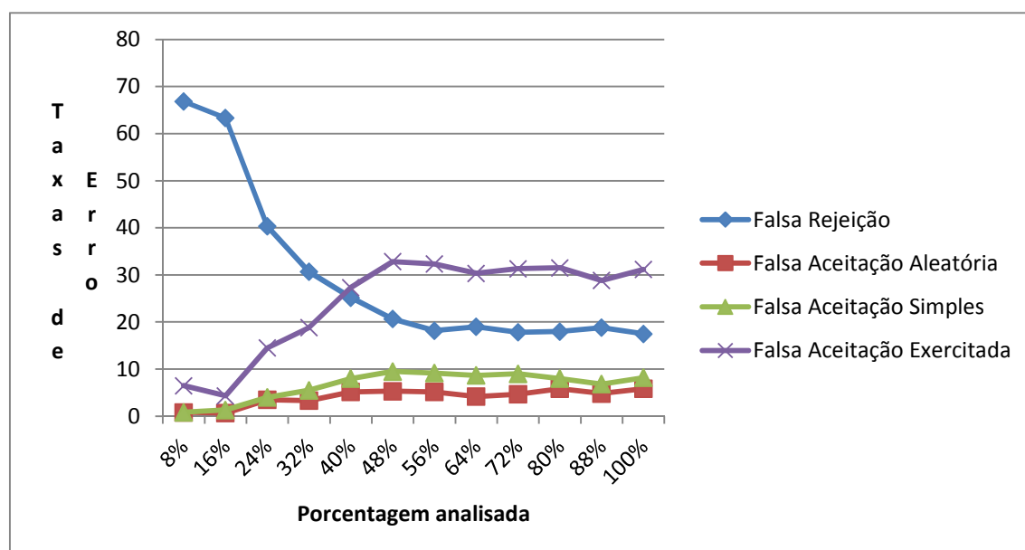
Figura 5.1: Gráfico das taxas de erro de acordo com a análise gradativa do grid .
