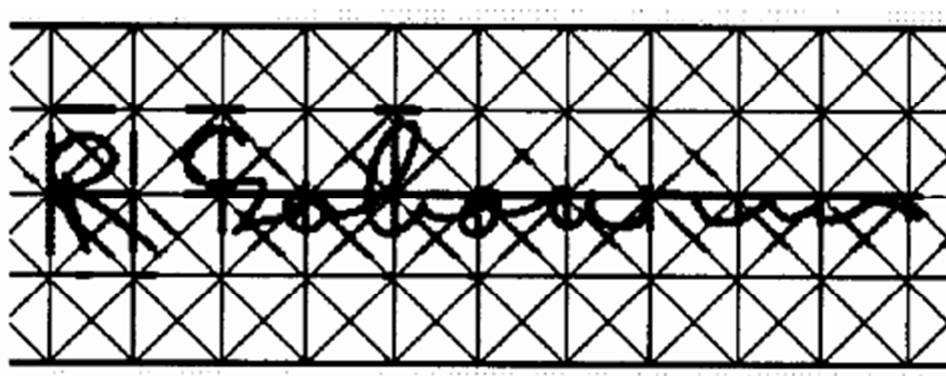
Figura 2.9: Modelo de célula utilizado por Sabourin e Genest. [JUSTINO, 2001]
