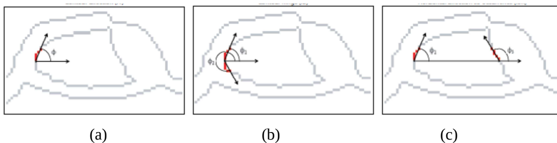
Figura 3.1: Descrição gráfica da extração de características. Onde (a) é a direção do contorno, (b) é a articulação do contorno e (c) é a co-ocorrência horizontal das direções. [GILPEREZ, 2008]
