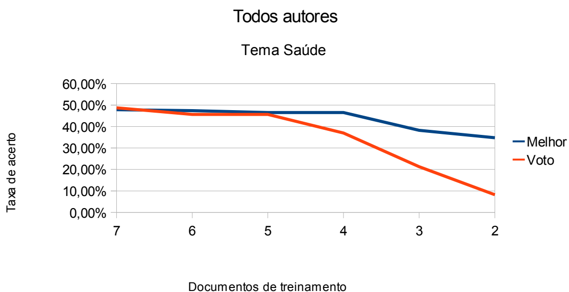
Figura 5.29: Taxa de acerto com diferentes quantidades de documentos de treinamento, compressor BZIP
