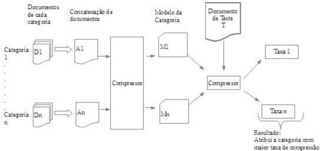
Figura 3.1: Procedimento SMDL
