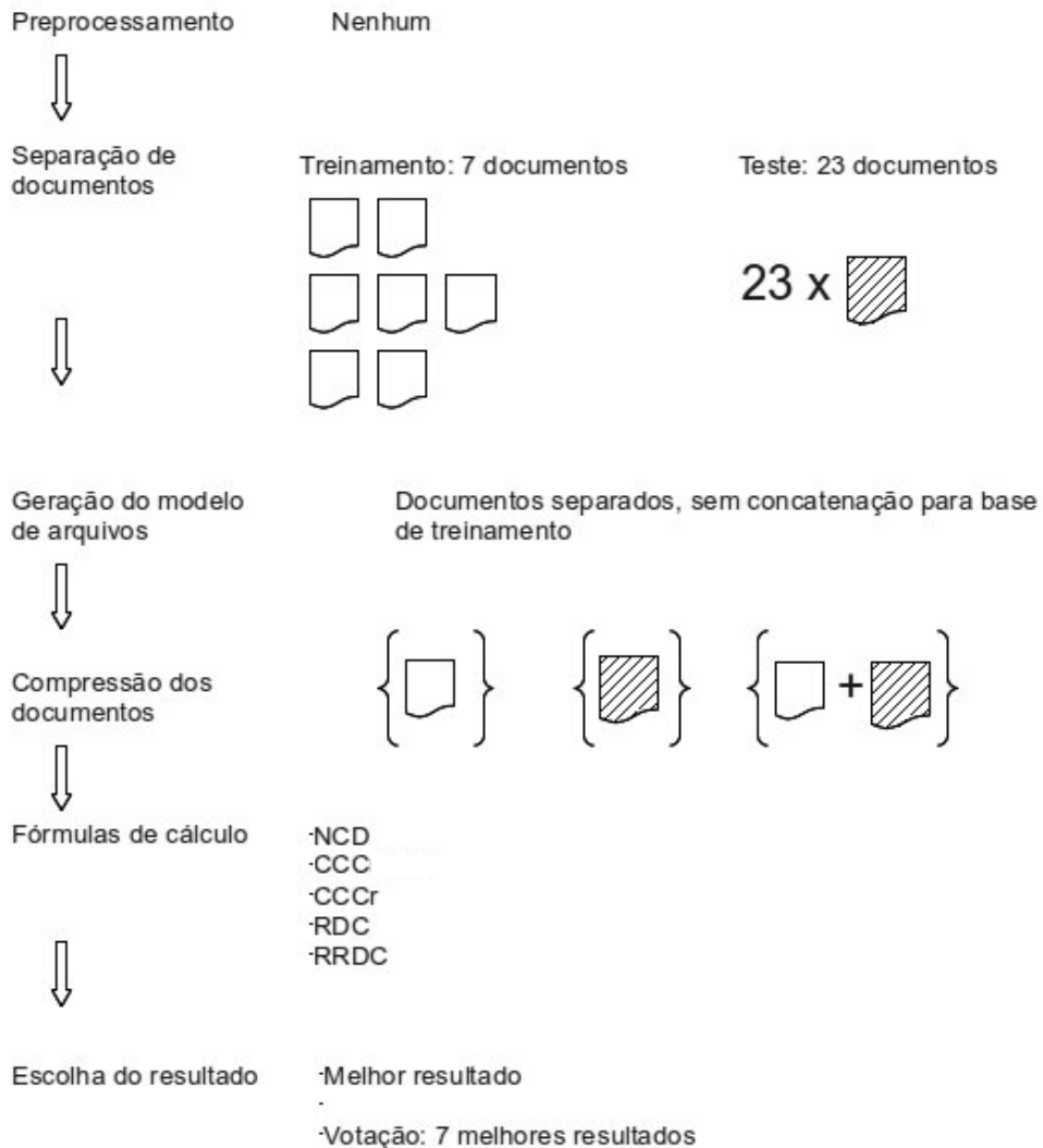
Figura 5.16: Procedimento de teste com documentos de treinamento individuais
