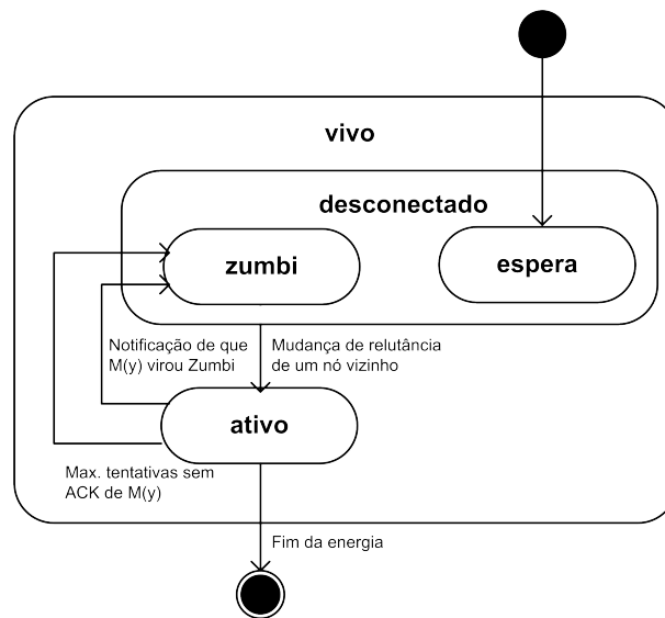
Figura 3.4: Diagrama de estados de um nó da rede
