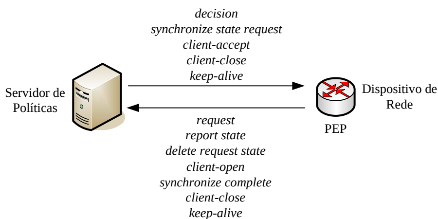
Figura 4.4: Protocolo COPS
