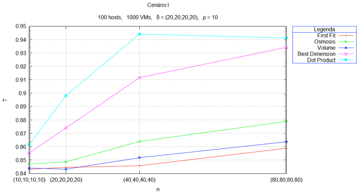
Figura 12. Gráfico para a taxa de alocação obtido no Cenário I.
