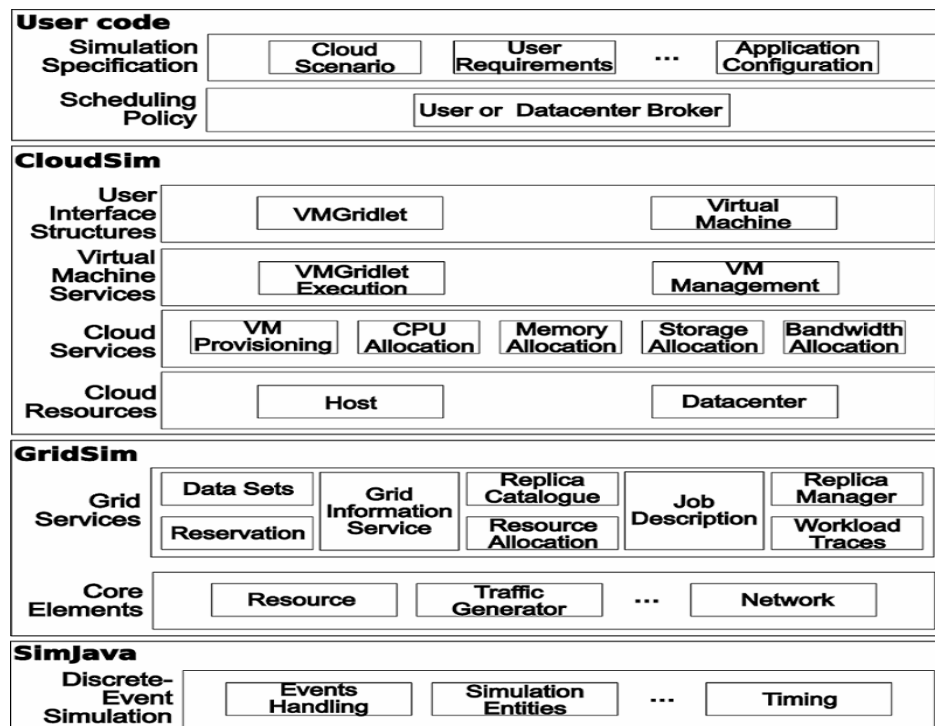
Figura 23. A arquitetura do CloudSim [Calheiros et al., 2010].
