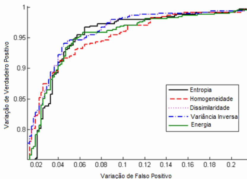
Figura 22. Curvas ROC comparando os descritores para dois níveis de cinza.
