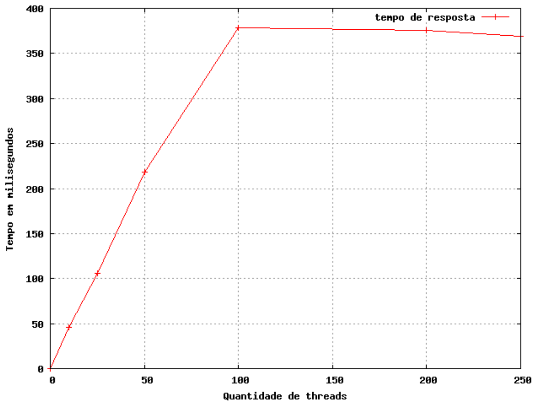
Figura 6.3: Impacto do número de threads na resposta do PDP
