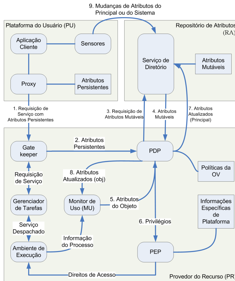
Figura 3.1: Arquitetura de autorização baseada em uso (ZHANG et al., 2006)
