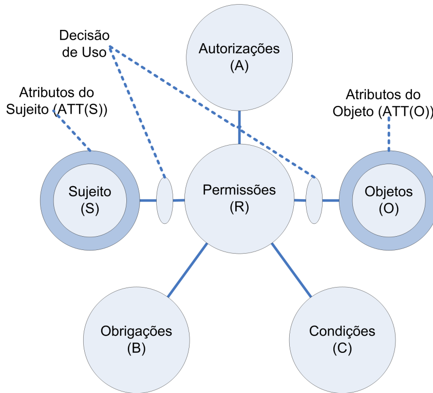
Figura 2.2: Componentes do UCON_{ABC} (PARK; SANDHU, 2004)
