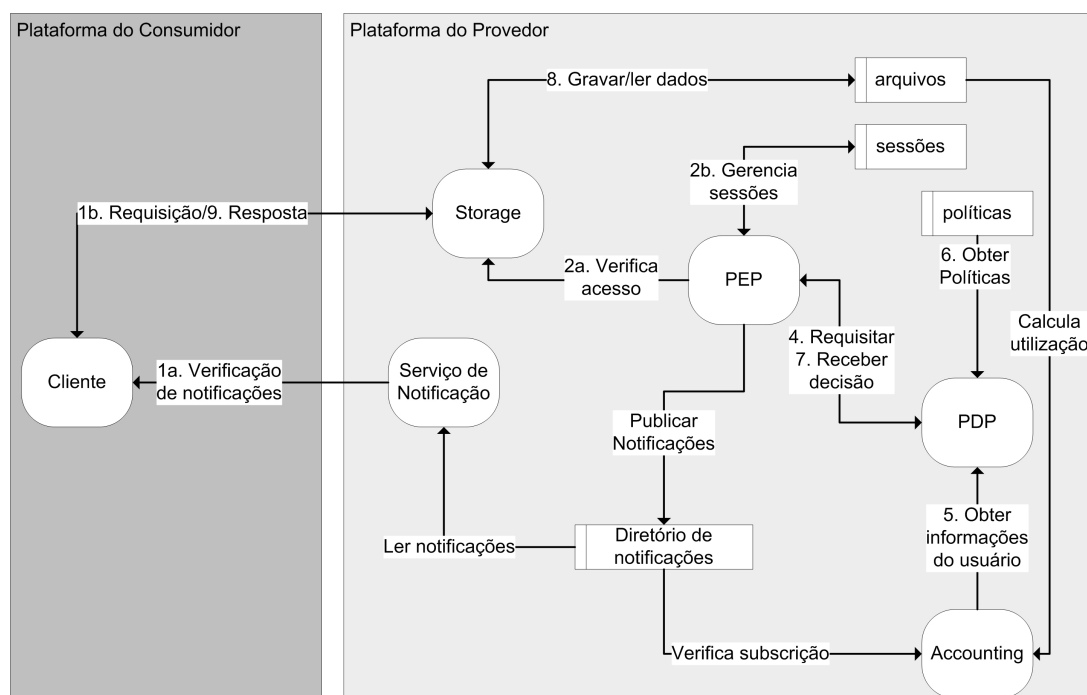
Figura 5.3: Visão geral das entidades do protótipo
