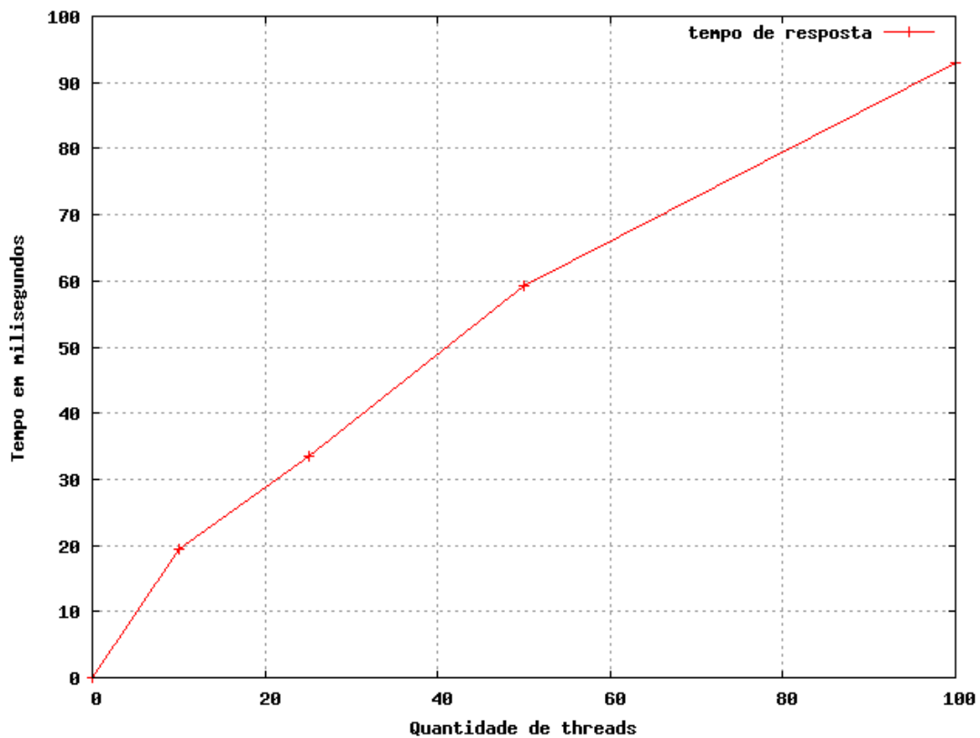
Figura 6.4: Impacto do número de threads na resposta do serviço de Accounting
