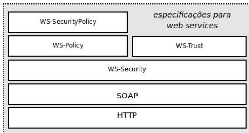
Figura 5.1: Protocolos e especificações para serviços web
