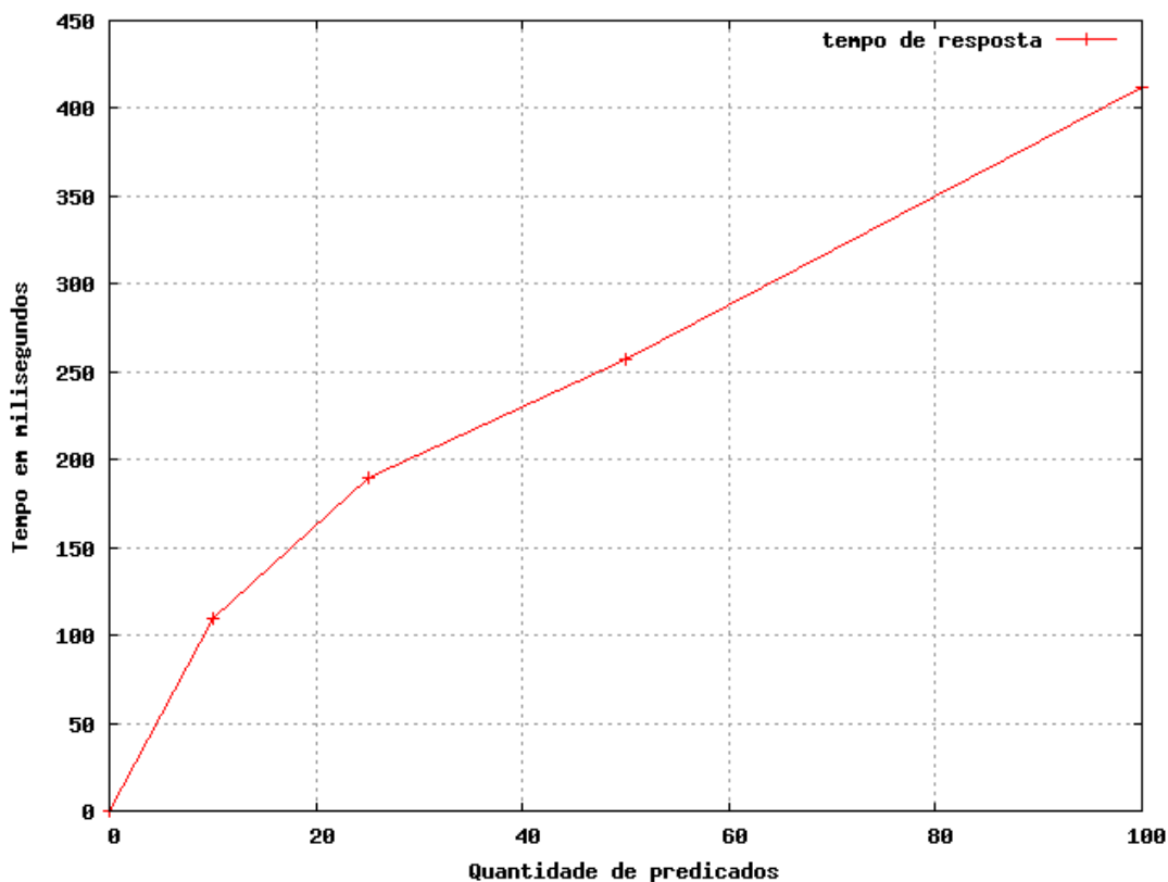
Figura 6.2: Impacto do número de predicados
