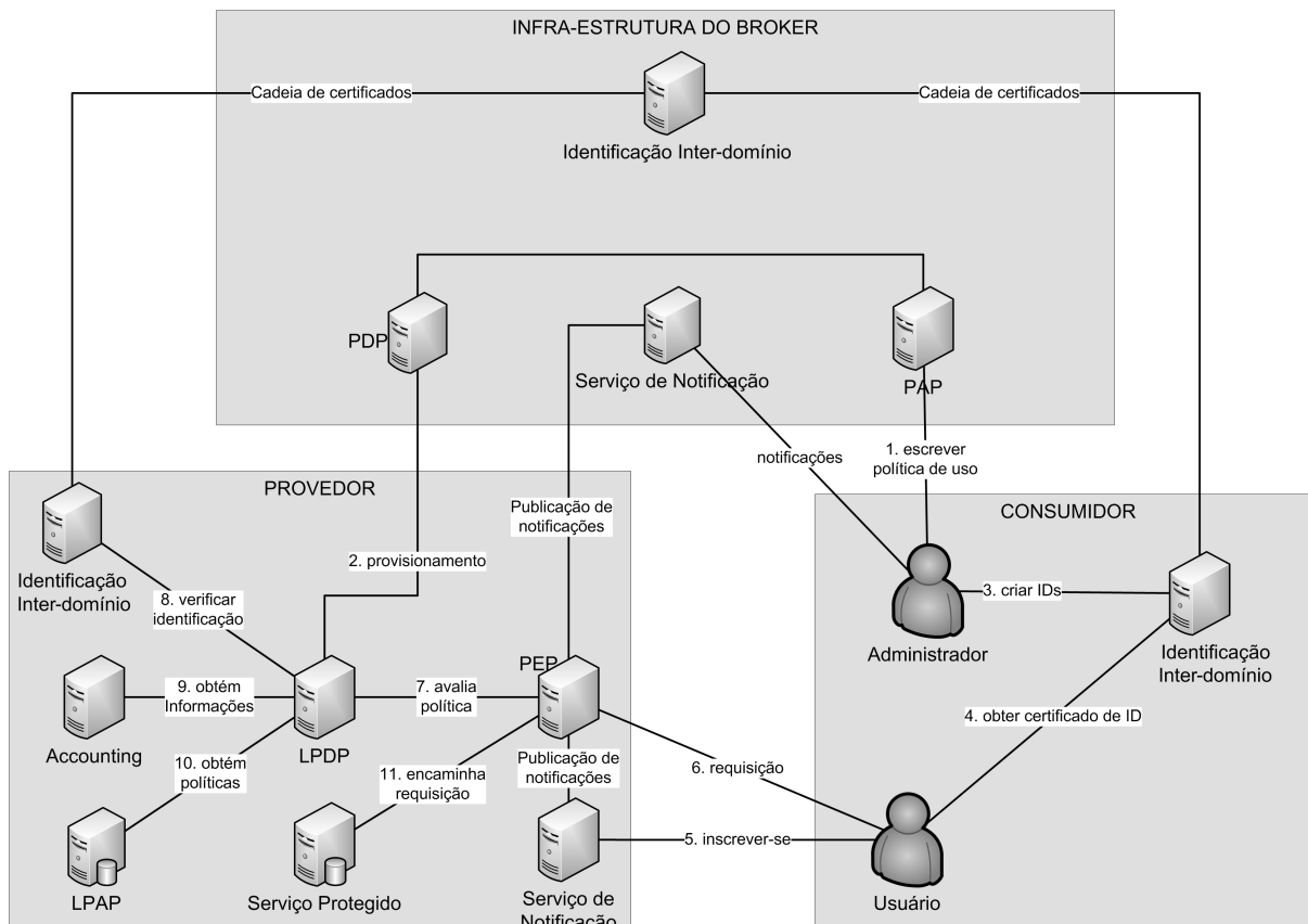
Figura 4.2: Visão geral da arquitetura proposta
