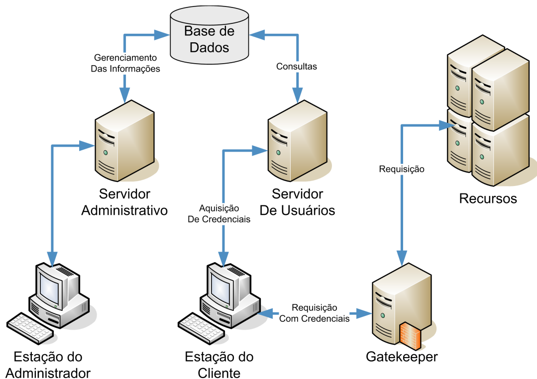
Figura 3.3: Visão conceitual do sistema VOMS
