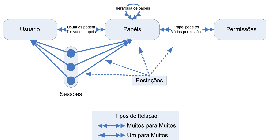
Figura 2.1: Elementos do modelo RBAC (SANDHU, 1998)
