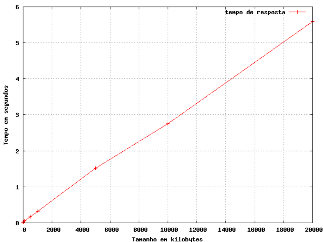
Figura 6.1: Impacto do tamanho dos pacotes no serviço de Storage
