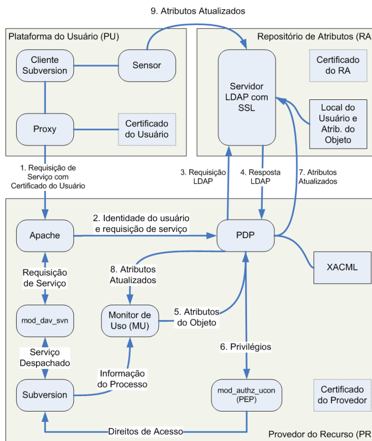
Figura 3.2: Arquitetura do protótipo (ZHANG et al., 2006)
