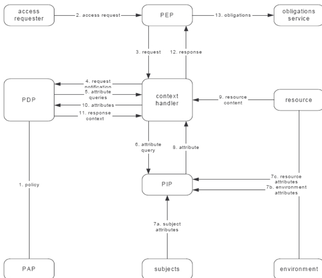
Figura 5.2: Fluxo de dados do modelo XACML (GODIK; MOSES, 2002)
