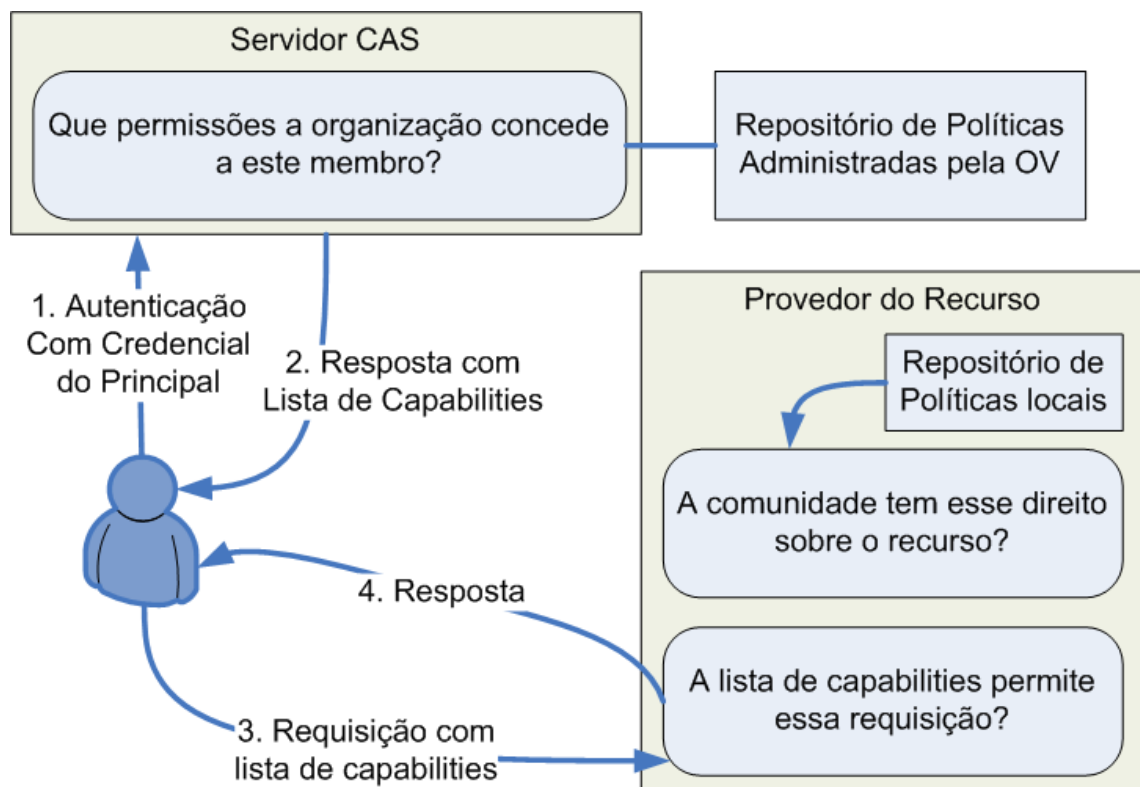
Figura 3.4: Visão conceitual do sistema CAS
