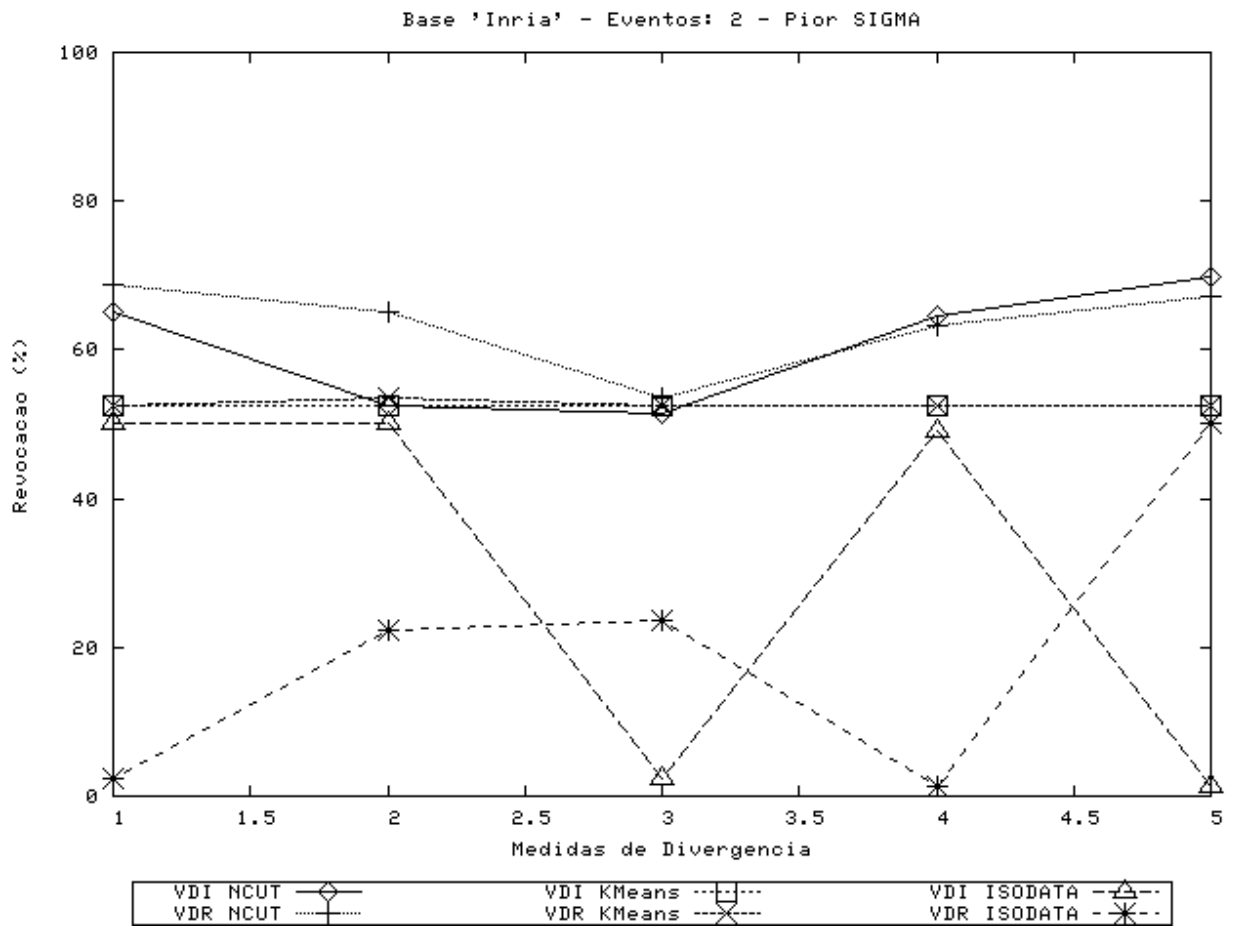
Figura A.16: Resultados de Revocação para vídeo “Inria”, 2 classes, pior caso, \sigma = 0, 10 .
