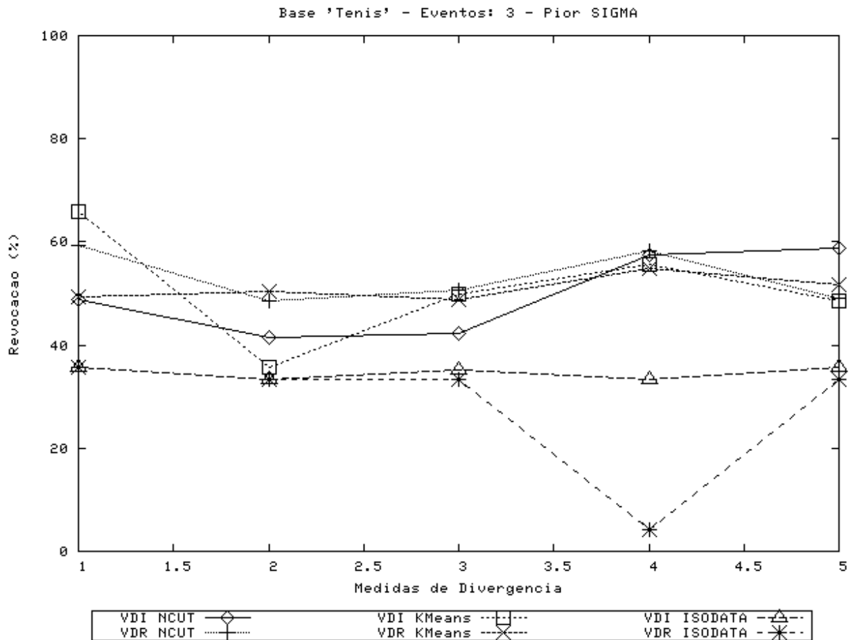
Figura A.4: Resultados de Revocação para vídeo “Tênis”, 3 classes, pior caso, \sigma = 0, 10 .
