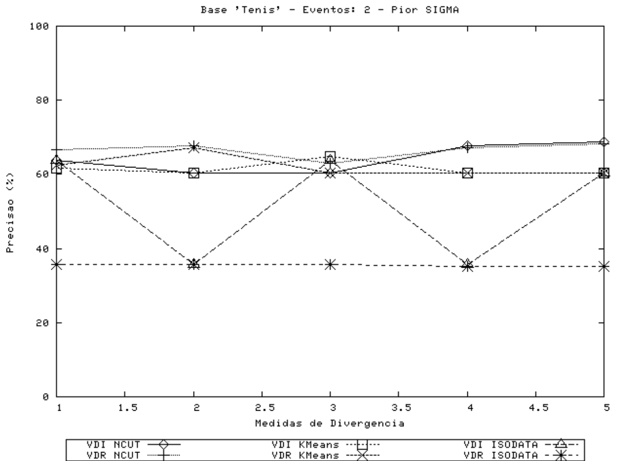
Figura A.7: Resultados de Precisão para vídeo “Tênis”, 2 classes, pior caso, \sigma = 0,60 .
