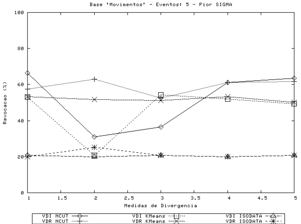
Figura 4.15: Resultados de Revocação para vídeo “Movimentos”, 5 classes, pior caso, \sigma = 0,95 .
