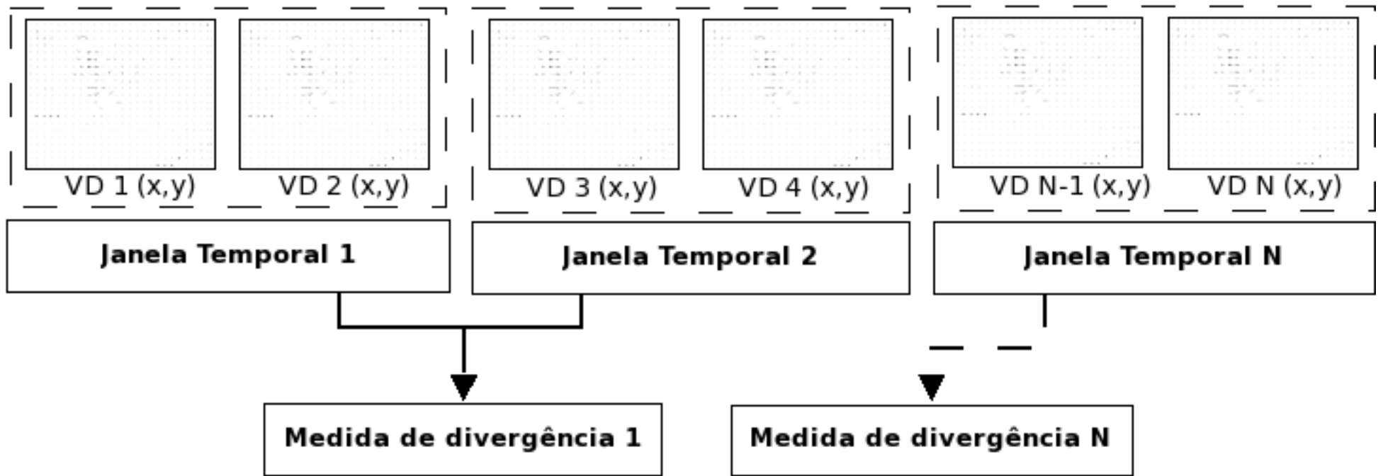
Figura 1.5: Aplicação de vetores de deslocamento em uma janela temporal de tamanho 2 para a geração de valores de divergência
