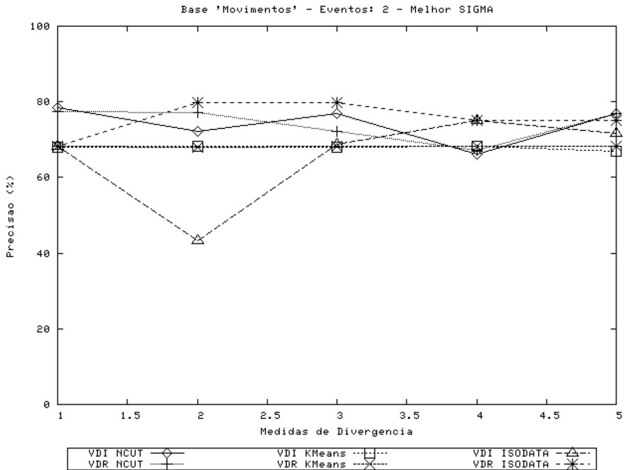
Figura 4.16: Resultados de Precisão para vídeo “Movimentos”, 2 classes, melhor caso, \sigma = 0,55 .
