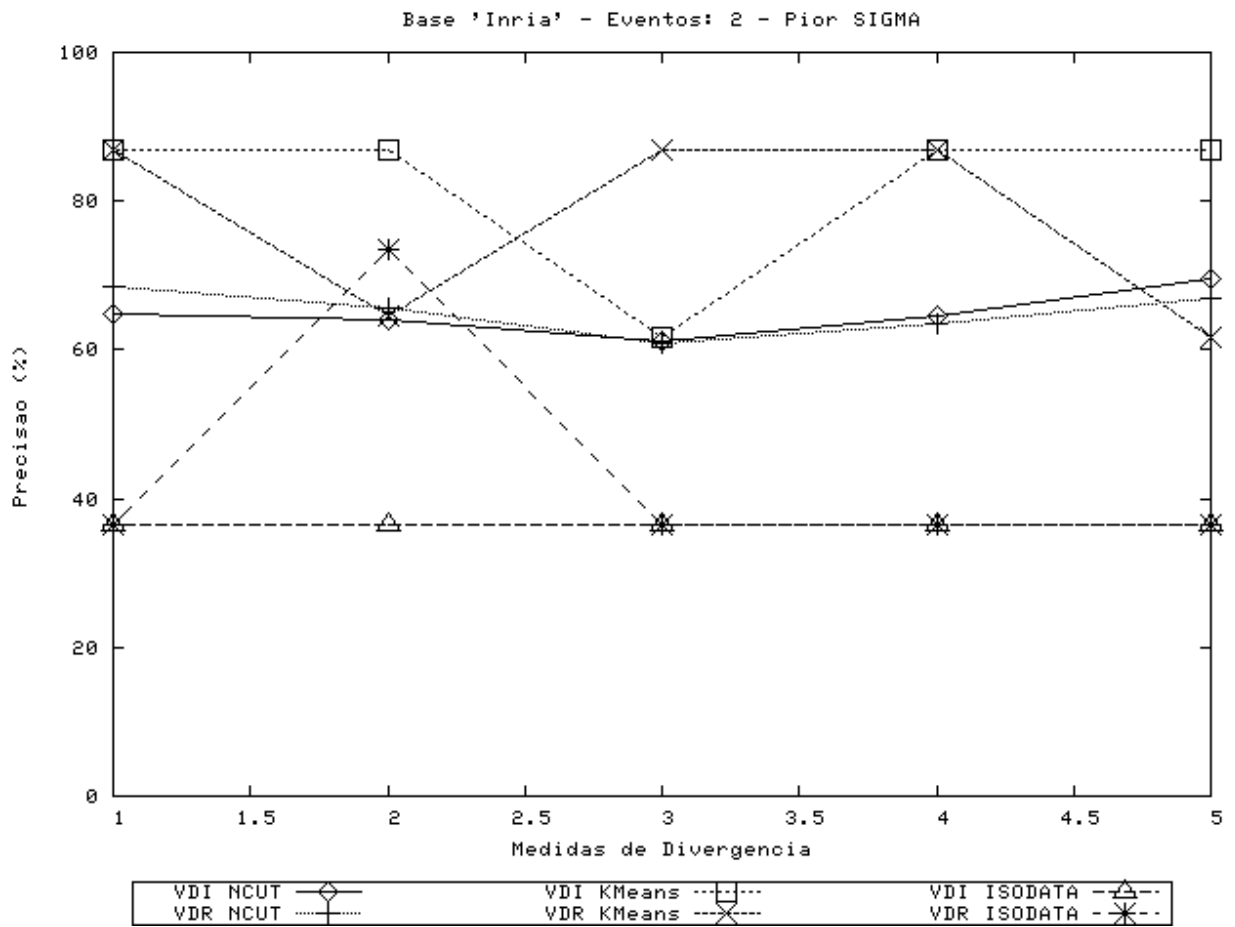
Figura A.15: Resultados de Precisão para vídeo “Inria”, 2 classes, pior caso, \sigma = 0, 10 .
