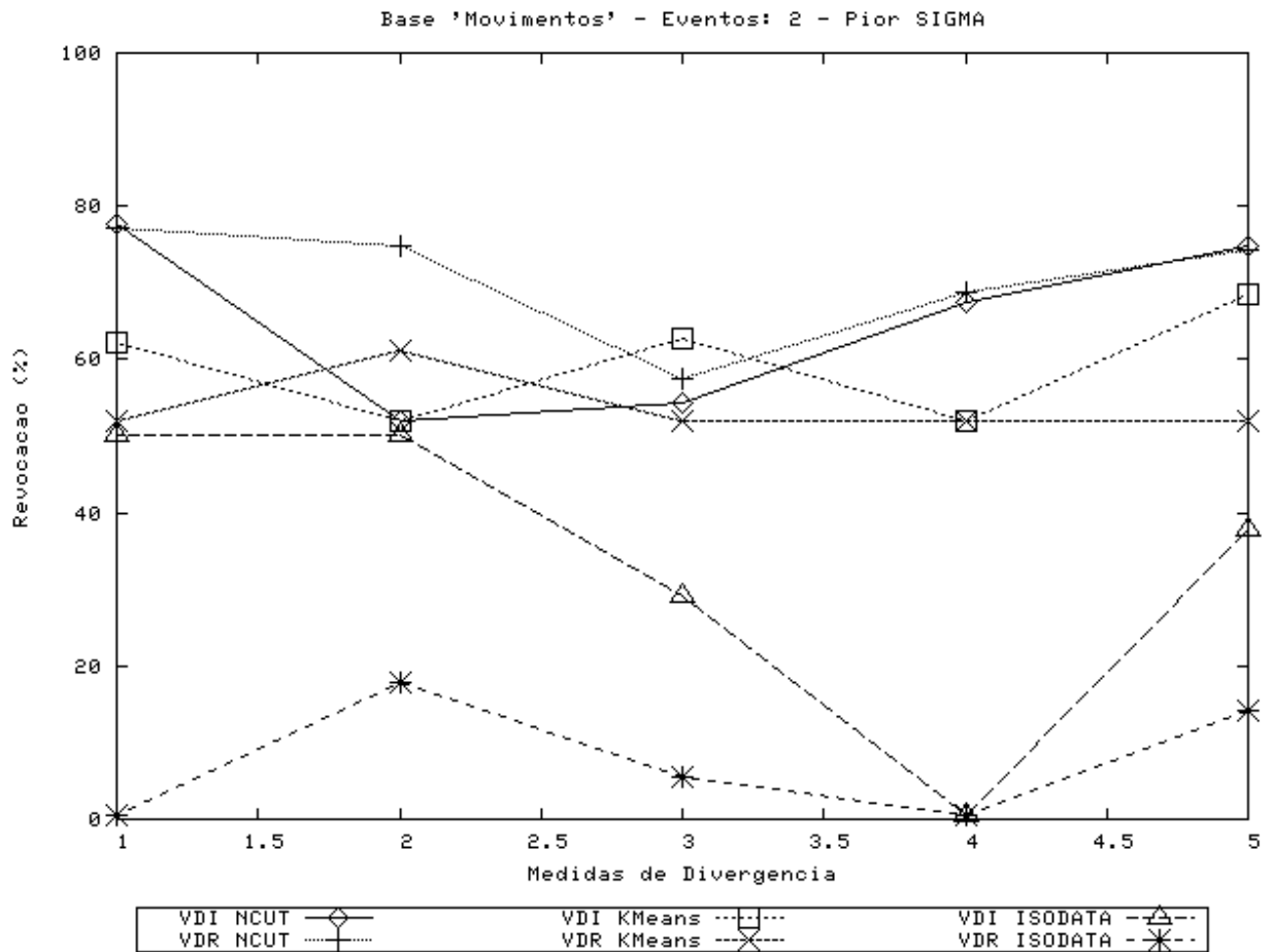
Figura 4.19: Resultados de Revocação para vídeo “Movimentos”, 2 classes, pior caso, \sigma = 0,85 .
