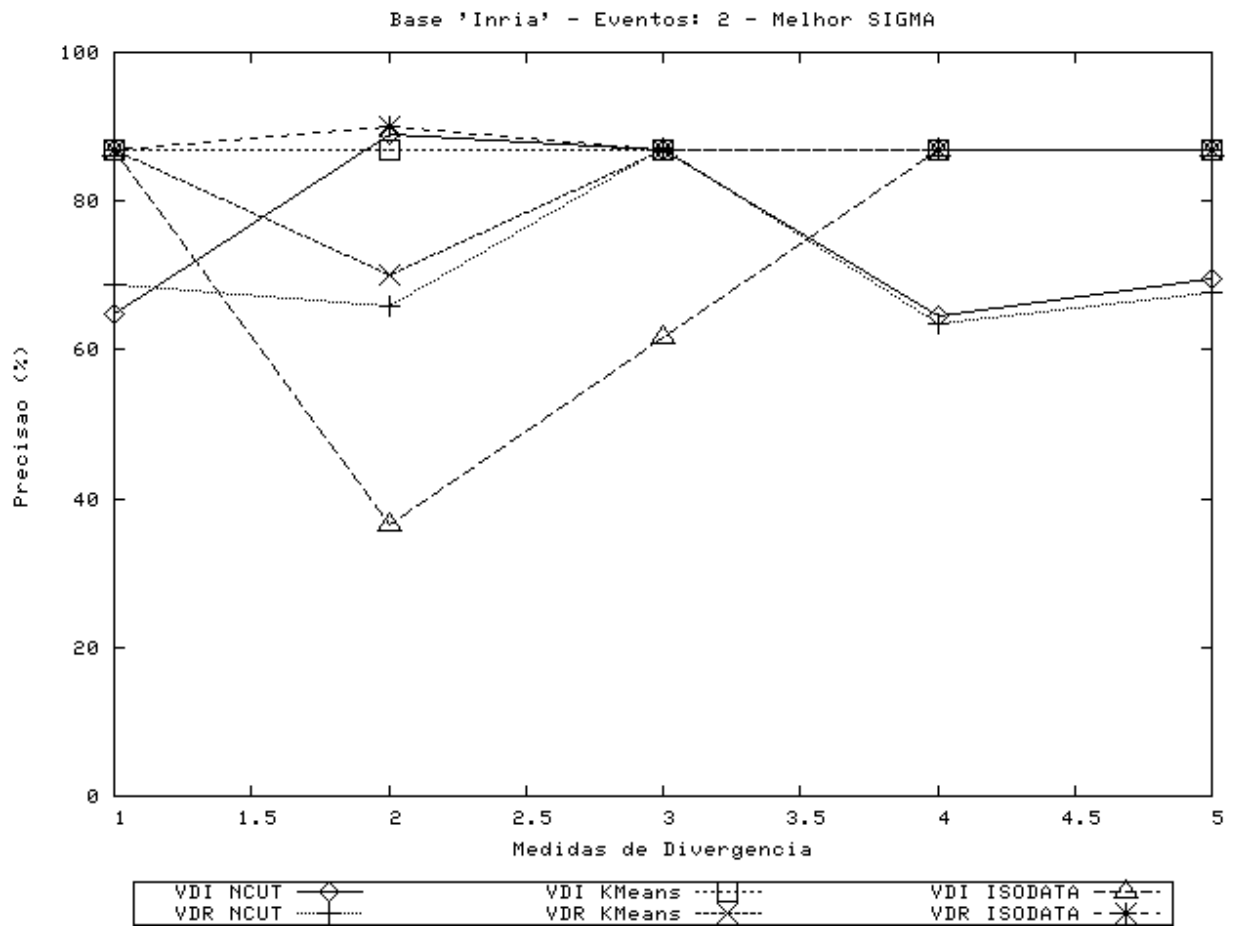
Figura A.13: Resultados de Precisão para vídeo “Inria”, 2 classes, melhor caso, \sigma = 0,05 .
