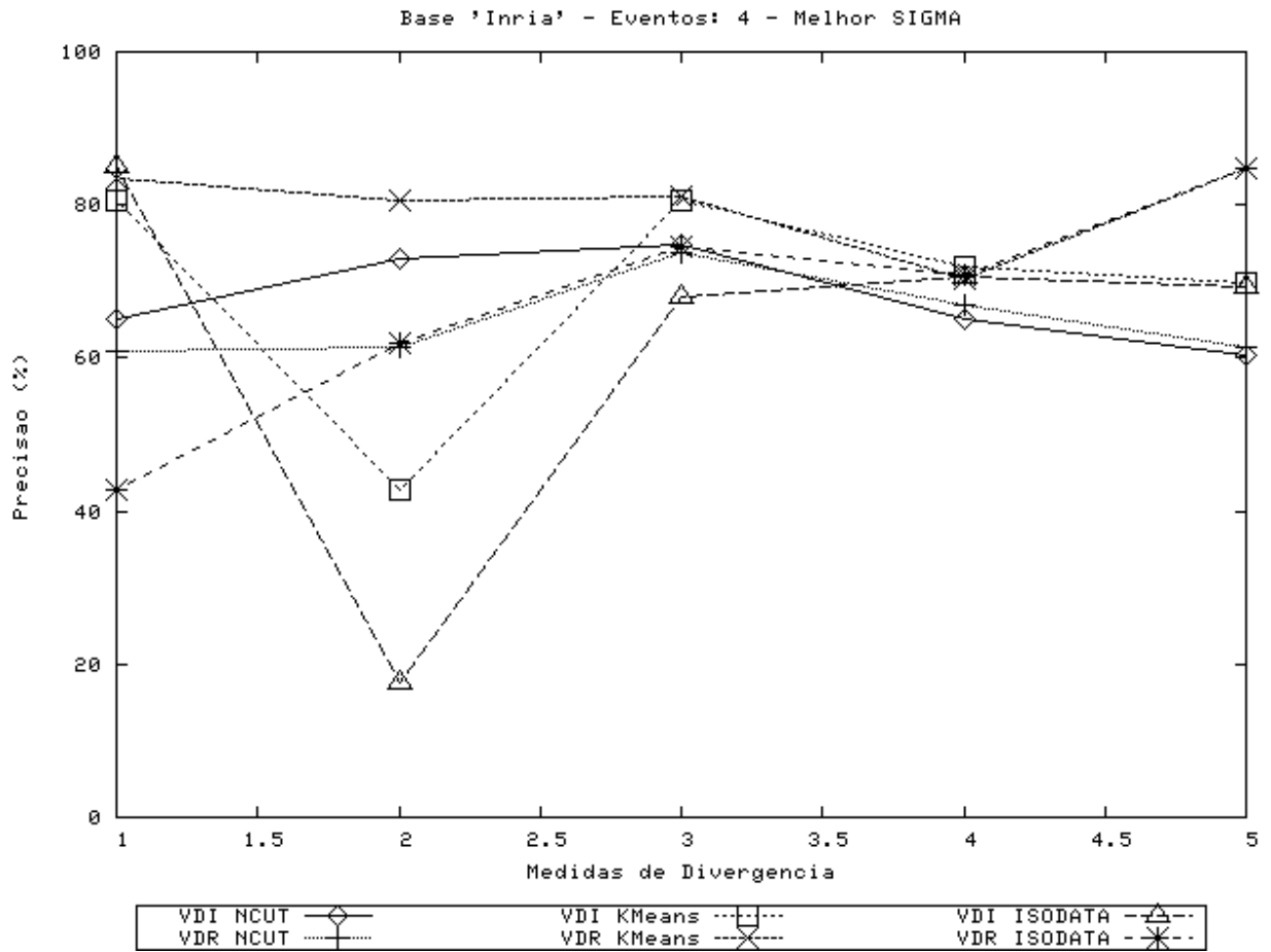
Figura A.9: Resultados de Precisão para vídeo “Inria”, 4 classes, melhor caso, \sigma = 0,85 .
