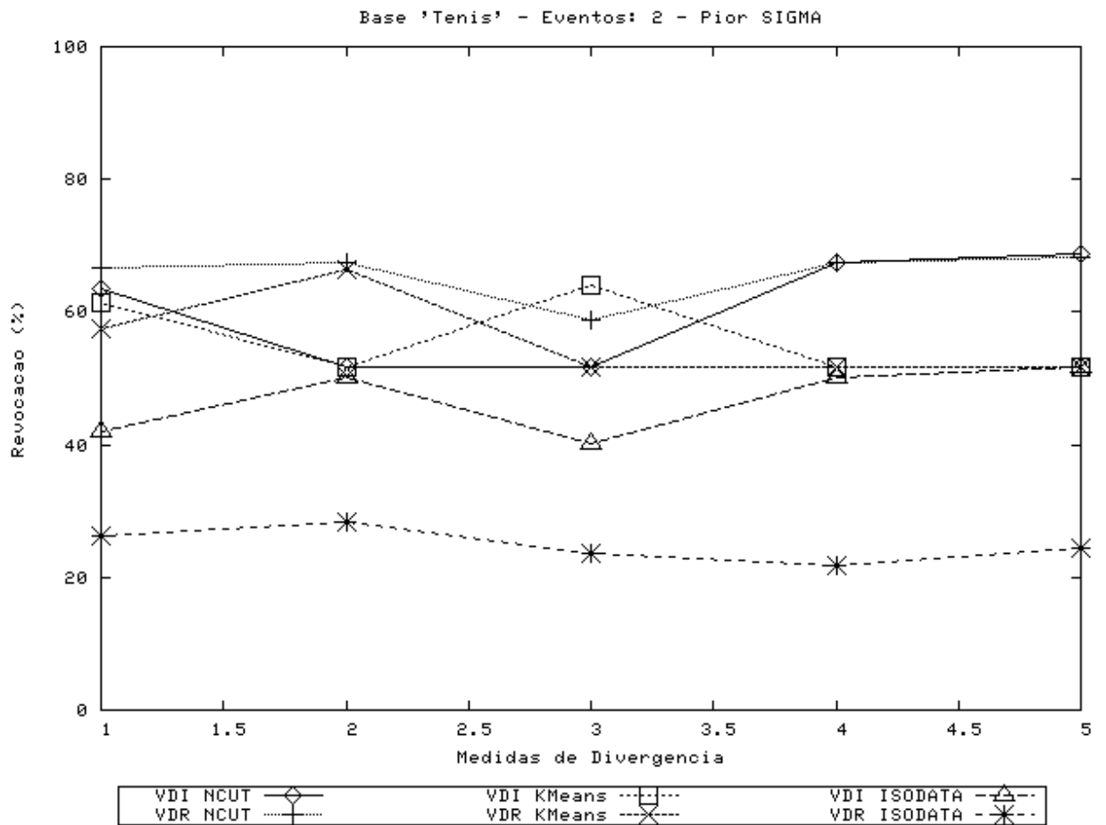
Figura A.8: Resultados de Revocação para vídeo “Tênis”, 2 classes, pior caso, \sigma = 0,60 .
