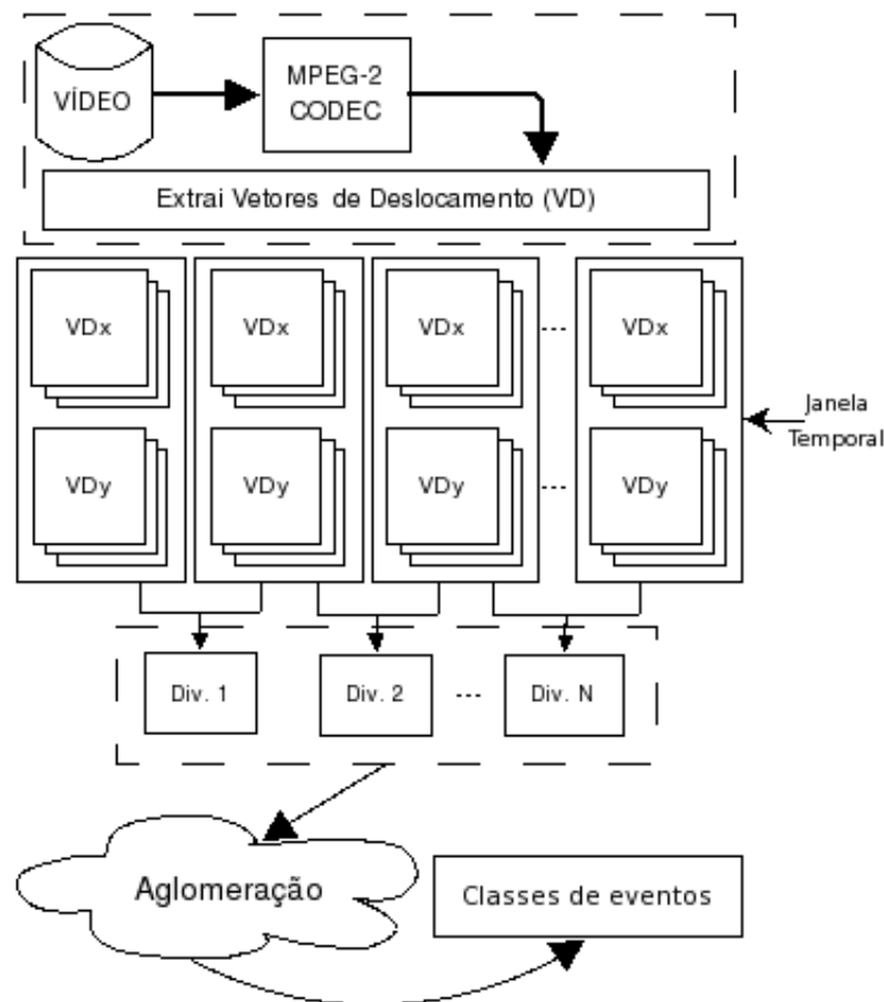
Figura 3.1: Diagrama de blocos do extrator de características. Vetores de deslocamento são extraídos para coordenadas x e y para cada janela temporal.
