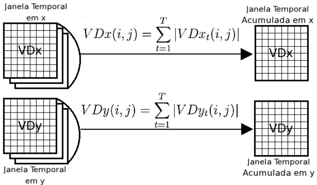
Figura 3.2: Diagrama que demonstra as características extraídas para cada janela temporal ( T ).
