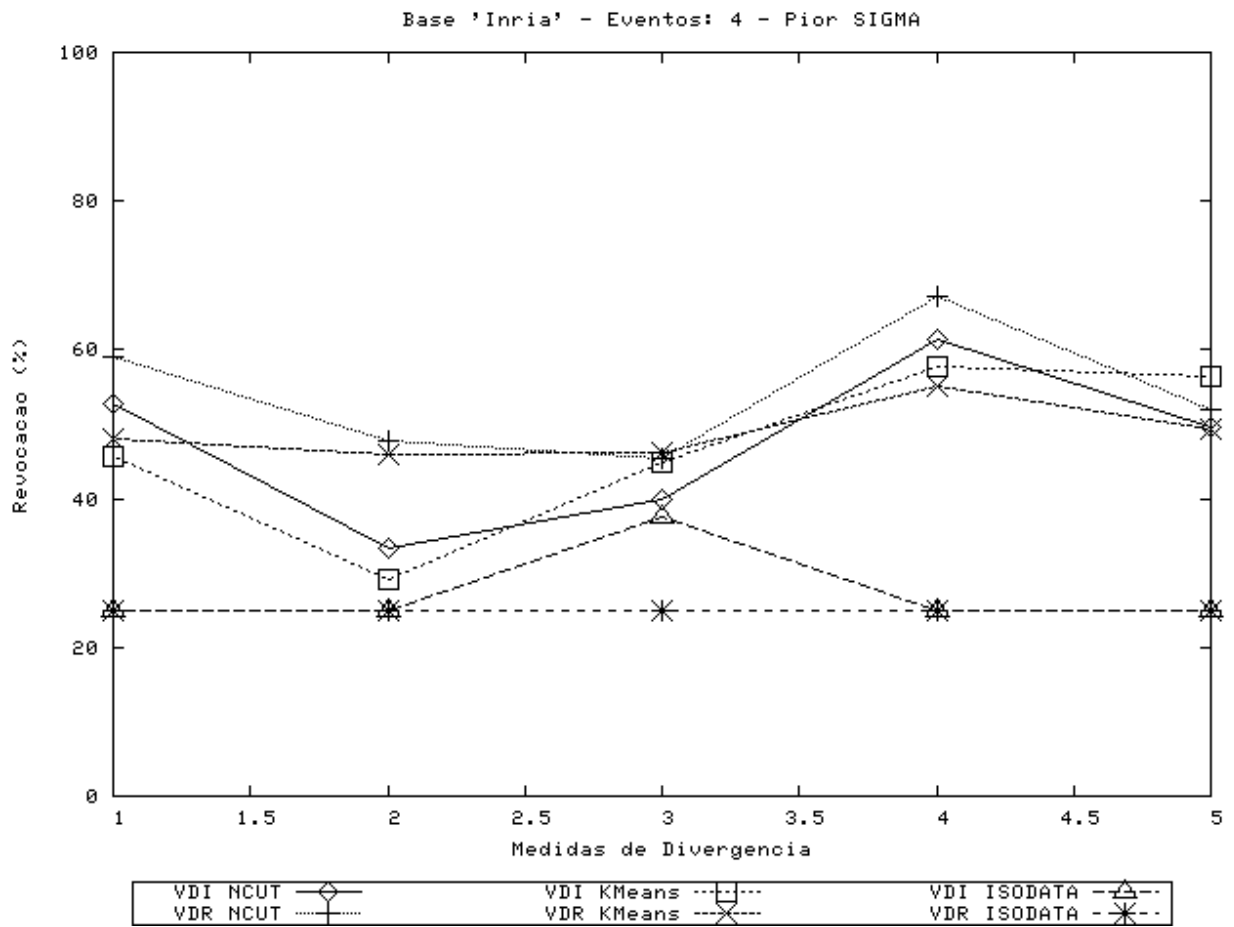
Figura A.12: Resultados de Revocação para vídeo “Inria”, 4 classes, pior caso, \sigma = 0,15 .
