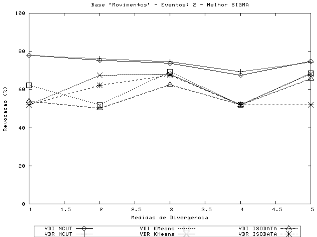
Figura 4.17: Resultados de Revocação para vídeo “Movimentos”, 2 classes, melhor caso, \sigma = 0,55 .
