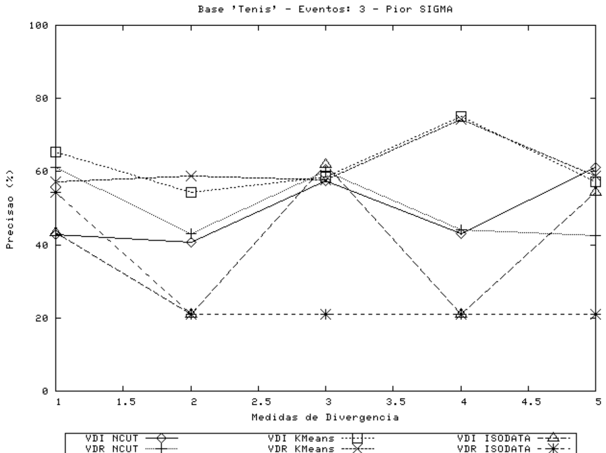
Figura A.3: Resultados de Precisão para vídeo “Tênis”, 3 classes, pior caso, \sigma = 0, 10 .
