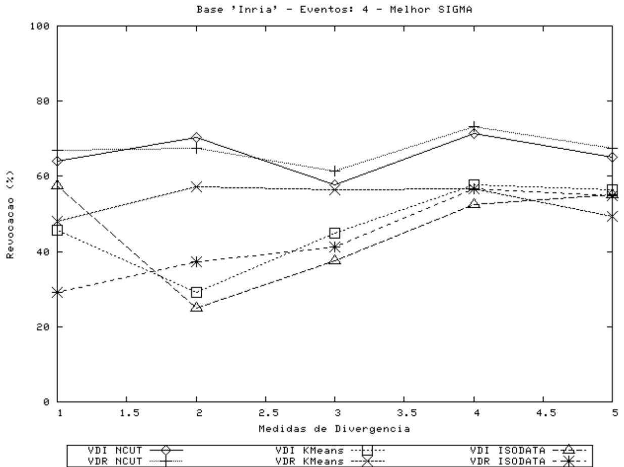
Figura A.10: Resultados de Revocação para vídeo “Inria”, 4 classes, melhor caso, \sigma = 0,85 .
