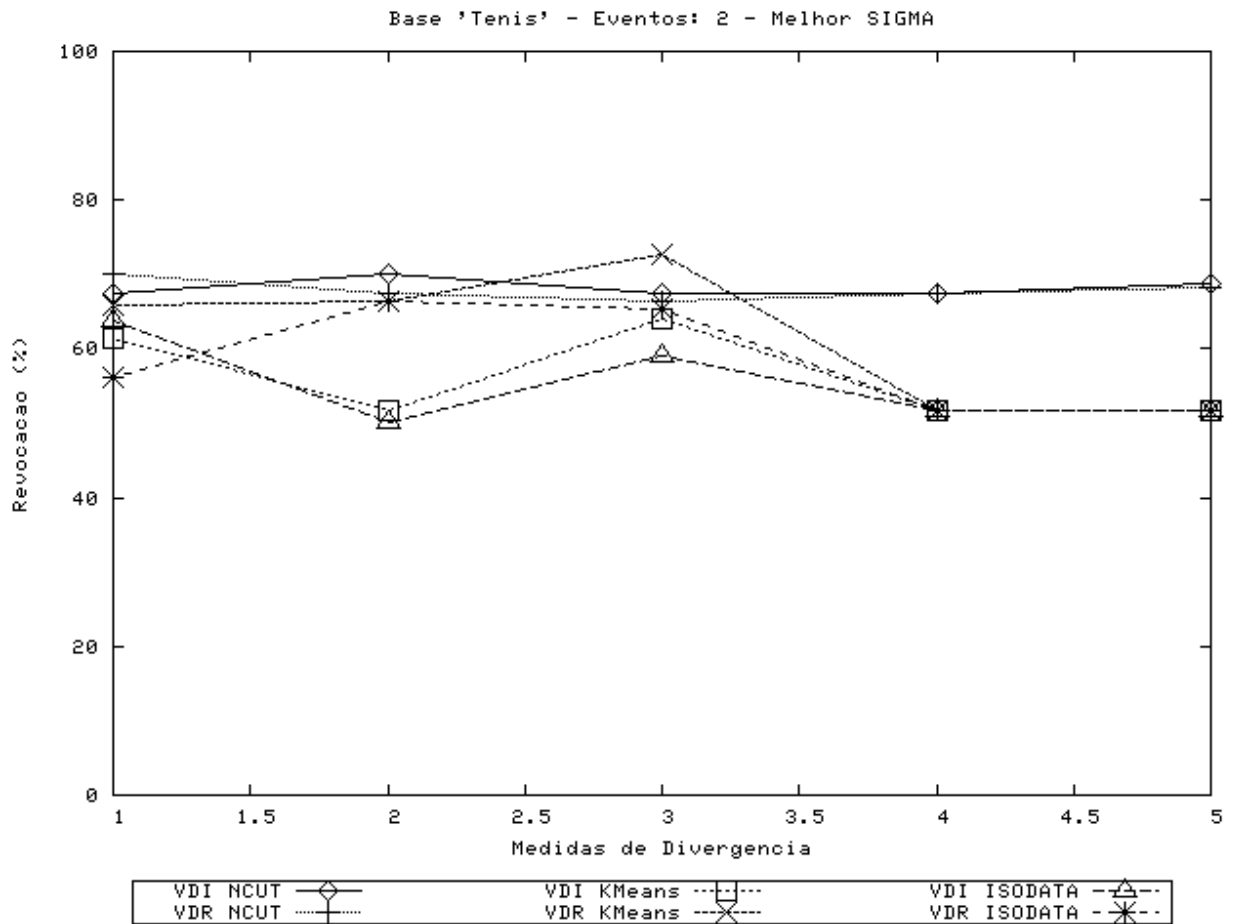
Figura A.6: Resultados de Revocação para vídeo “Tênis”, 2 classes, melhor caso, \sigma = 0,50 .
