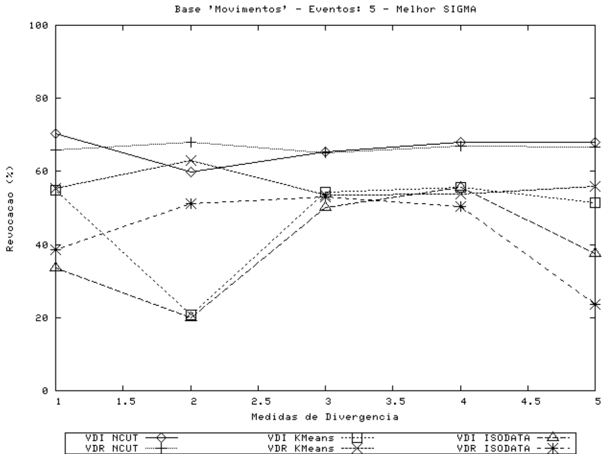
Figura 4.13: Resultados de Revocação para vídeo “Movimentos”, 5 classes, melhor caso, \sigma = 0,40 .
