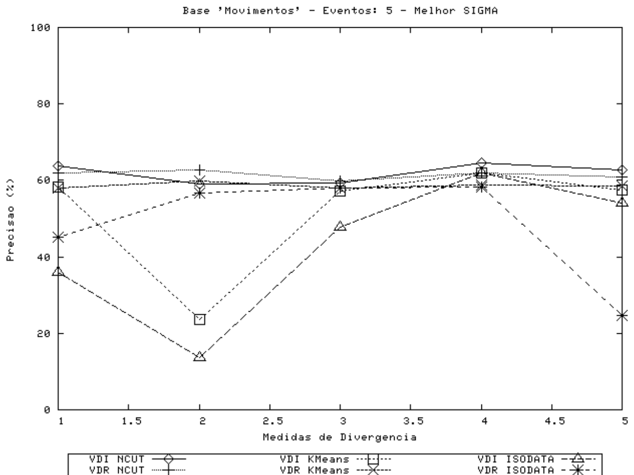
Figura 4.12: Resultados de Precisão para vídeo “Movimentos”, 5 classes, melhor caso, \sigma = 0, 40 .
