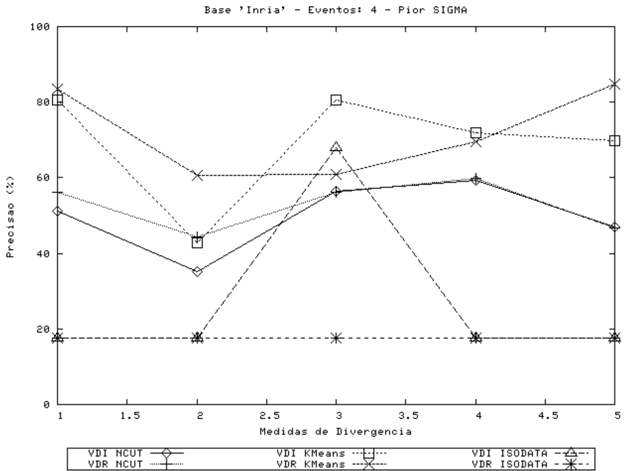
Figura A.11: Resultados de Precisão para vídeo “Inria”, 4 classes, pior caso, \sigma = 0,15 .
