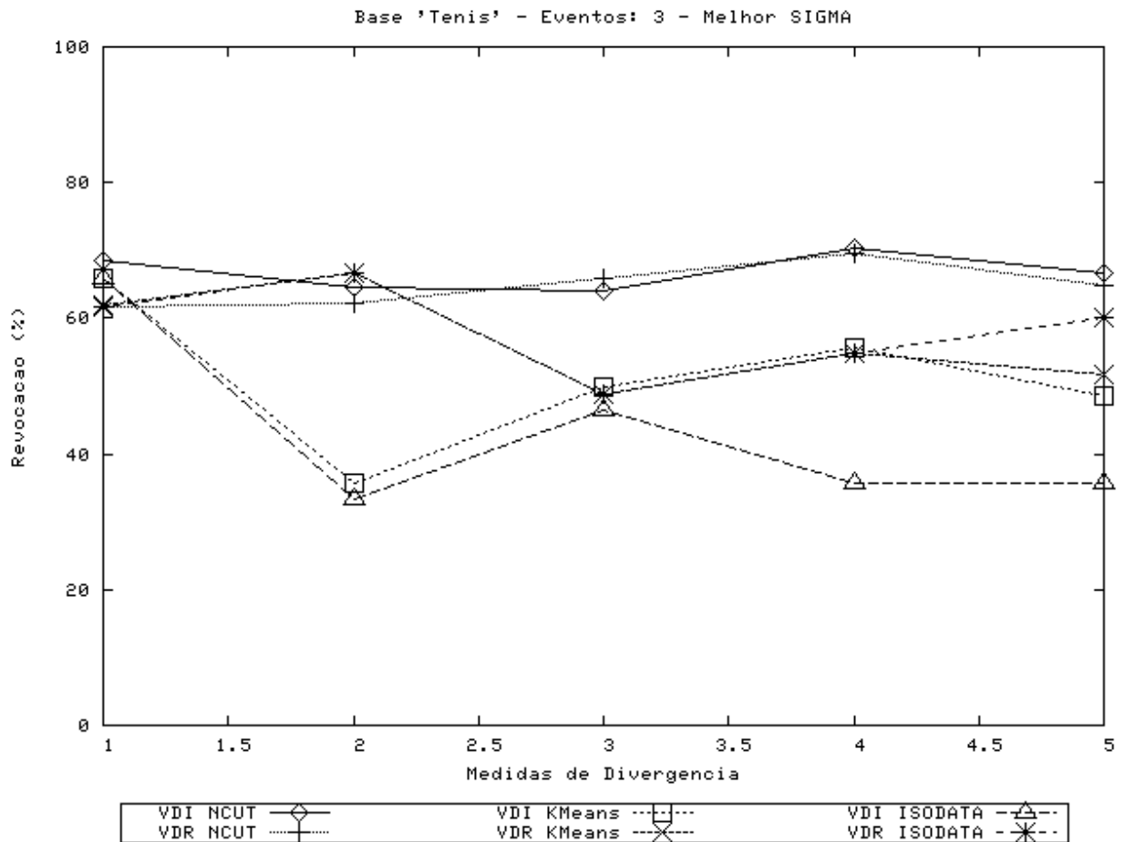
Figura A.2: Resultados de Revocação para vídeo “Tênis”, 3 classes, melhor caso, \sigma = 0,85 .
