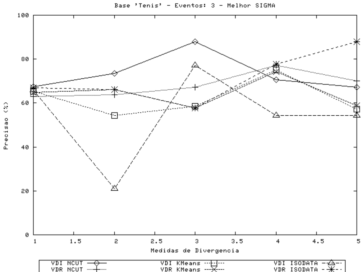
Figura A.1: Resultados de Precisão para vídeo “Tênis”, 3 classes, melhor caso, \sigma = 0,85 .
