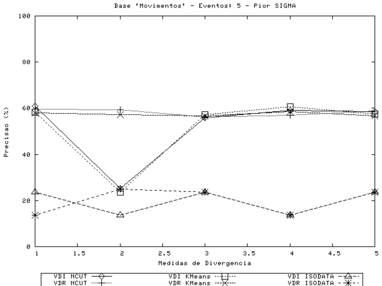
Figura 4.14: Resultados de Precisão para vídeo “Movimentos”, 5 classes, pior caso, \sigma = 0,95 .
