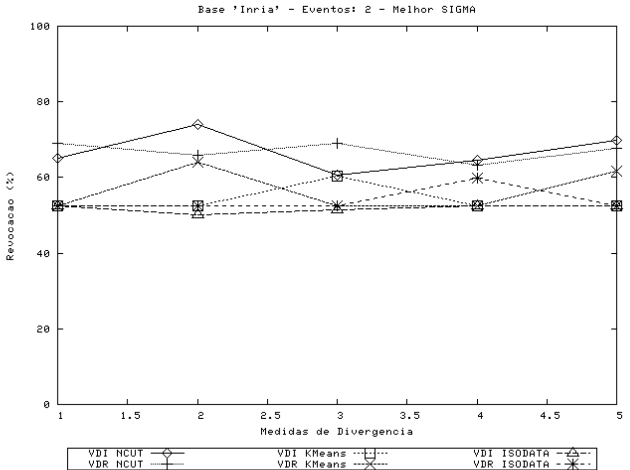
Figura A.14: Resultados de Revocação para vídeo “Inria”, 2 classes, melhor caso, \sigma = 0,05 .
