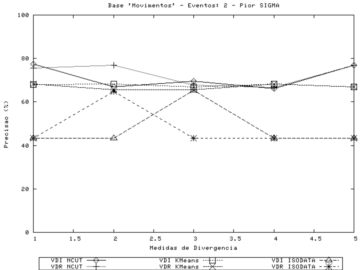
Figura 4.18: Resultados de Precisão para vídeo “Movimentos”, 2 classes, pior caso, \sigma = 0,85 .
