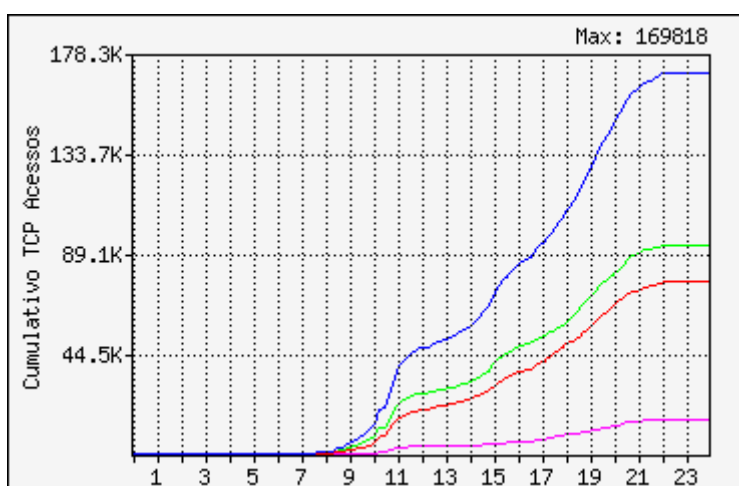
FIGURA 47 - GRÁFICO CUMULATIVO DE REQUISIÇÕES (HIT RATE) NO LOTE S-04-A.
