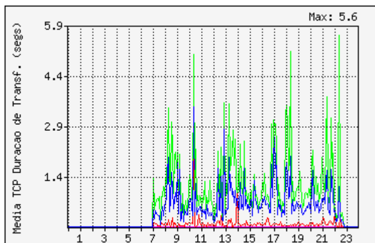
FIGURA 51 - GRÁFICO DE DURAÇÃO MÉDIA DE TRANSFERÊNCIA (LATÊNCIA) NO LOTE S-05-A.
