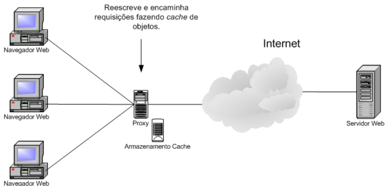
FIGURA 3 - PROXY UTILIZADO EM UMA COMUNICAÇÃO COM O PROTOCOLO HTTP.
