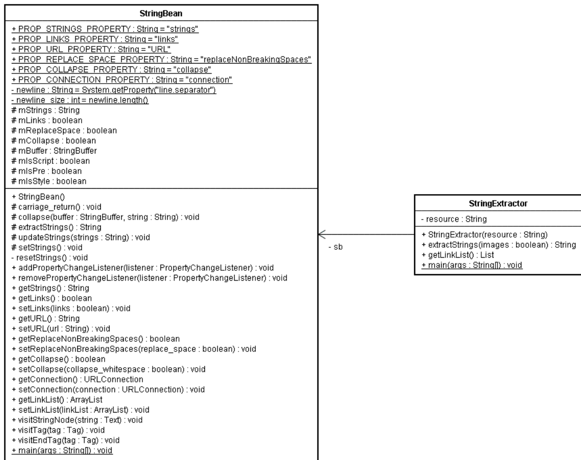
FIGURA 32 - DIAGRAMA DE CLASSES DO PACOTE HTML .
