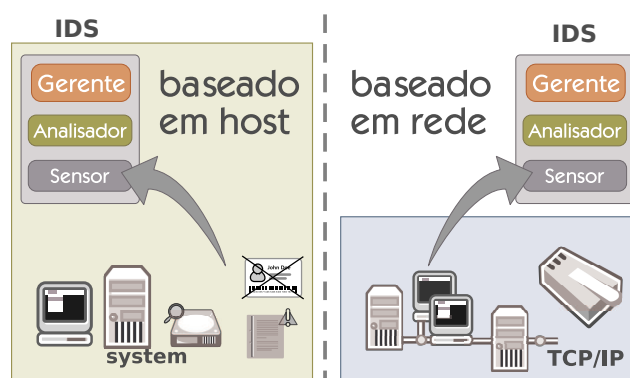
Figura 2.2: Ilustração - IDS baseado em Hospedeiro e IDS baseado em Rede
