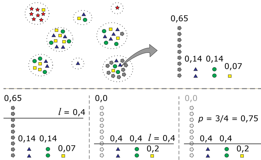
Figura 4.7: Ilustração - Cálculo do índice de popularidade
