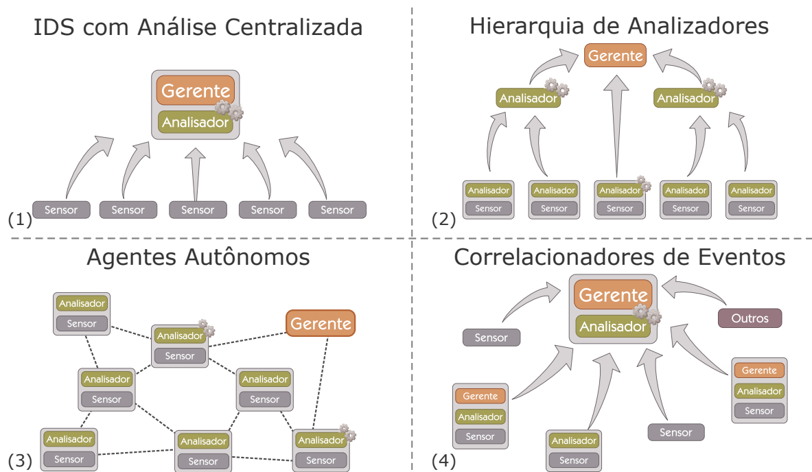
Figura 2.9: Ilustração - Arquiteturas de IDSs Distribuídos
