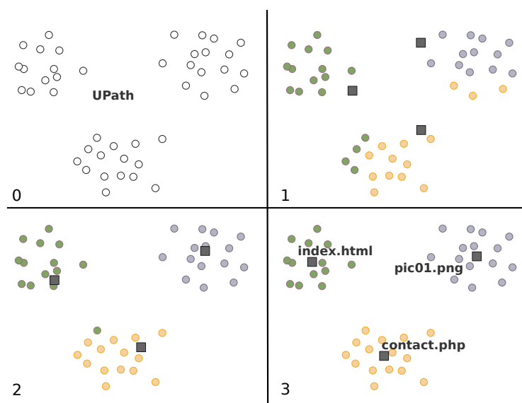
Figura 4.5: Ilustração - Agrupamento K-Means em 3 iterações
