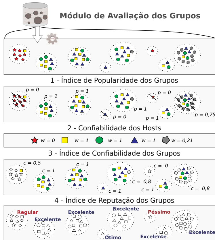
Figura 4.6: Ilustração - As quatro etapas para avaliação dos grupos
