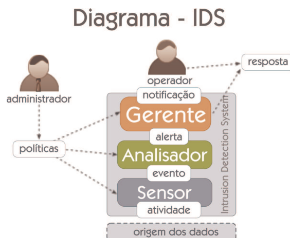
Figura 2.1: Diagrama de IDS - RFC 4766
