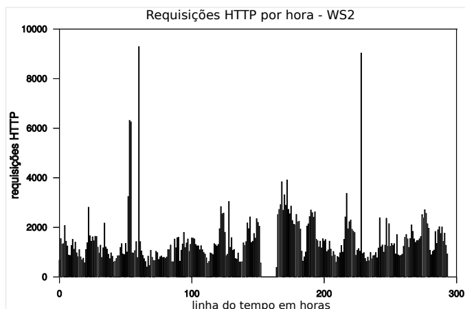
Figura 5.2: Gráfico - Requisições HTTP de WS2
