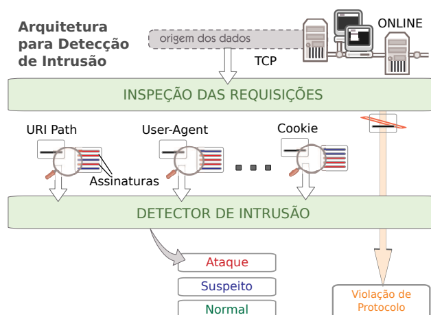
Figura 4.11: Ilustração - Arquitetura para Detecção de Intrusão
