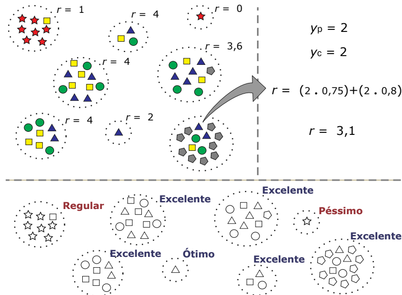
Figura 4.10: Ilustração - Cálculo do índice de reputação
