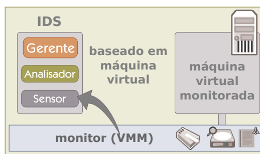
Figura 2.3: Ilustração - IDS baseado em Máquina Virtual
