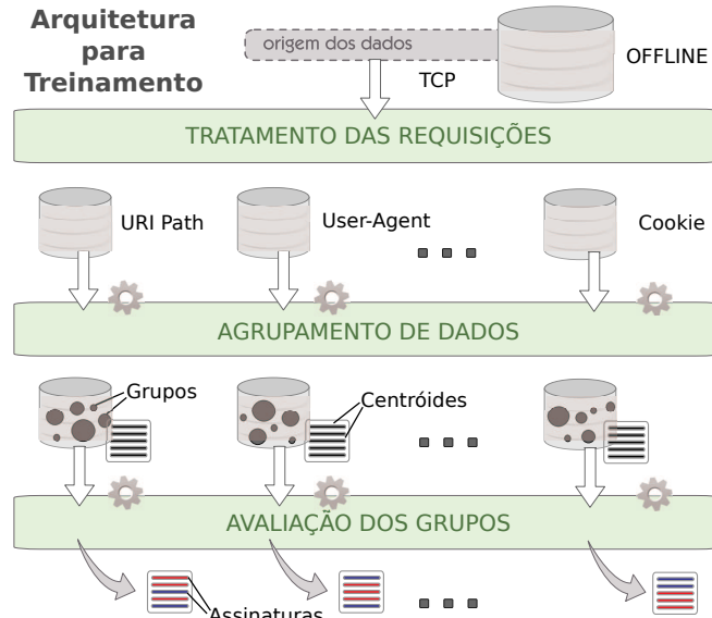
Figura 4.1: Ilustração - Arquitetura para treinamento
