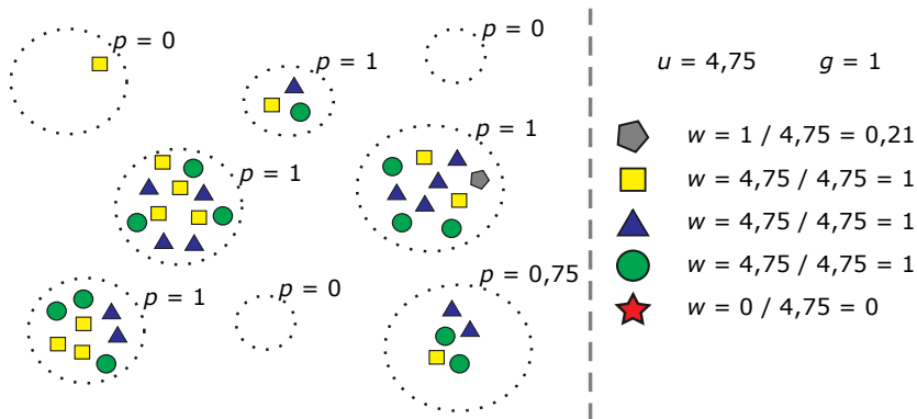
Figura 4.8: Ilustração - Cálculo da confiabilidade dos hosts
