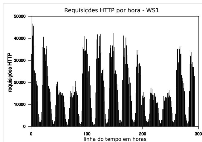
Figura 5.1: Gráfico - Requisições HTTP de WS1
