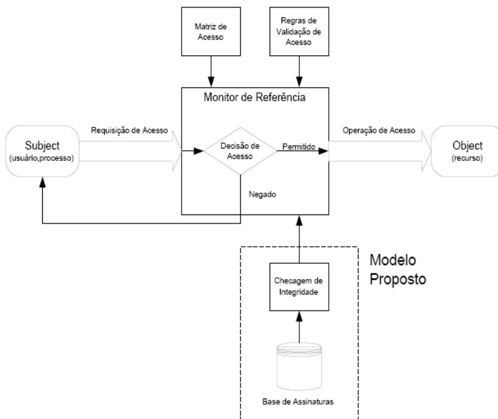
Figura 3.5. – Representação do Monitor de Referência com a incorporação do Modelo Proposto [BOR01]
