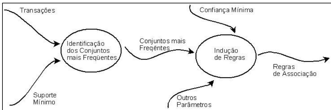
Figura 5.3: Estrutura do Programa APriori [SOU00]
