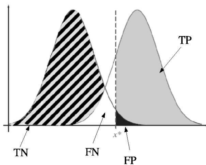
Figura 23: Impacto da escolha de um ponto operacional nas taxas de TP, FP, TN e FN.
