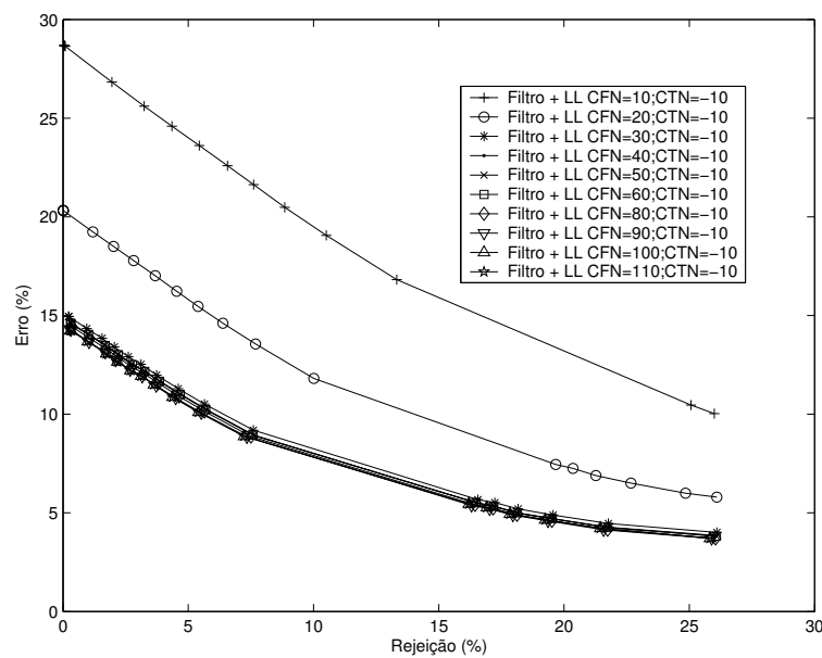
Figura 32: Taxas de reconhecimento de cadeias de caracteres utilizando o filtro proposto + low level aliado aos esquemas de custo da Tabela 3.
