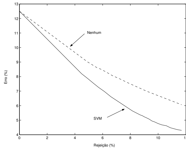
Figura 27: Impacto do método proposto em termos de taxa de erro versus taxa de rejeição.
