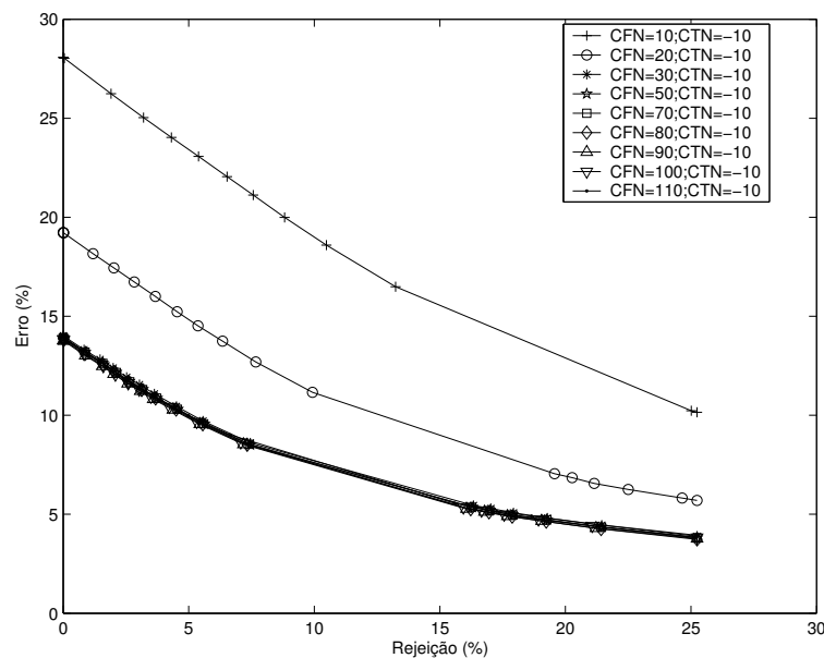
Figura 31: Taxas de reconhecimento de cadeias de caracteres utilizando o filtro proposto aliado aos esquemas de custo da Tabela 3.
