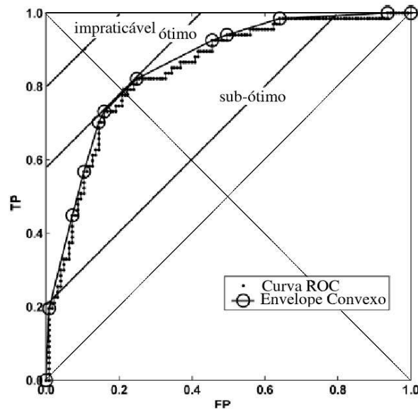
Figura 13: Mecanismo de custo iso-performance [21]
