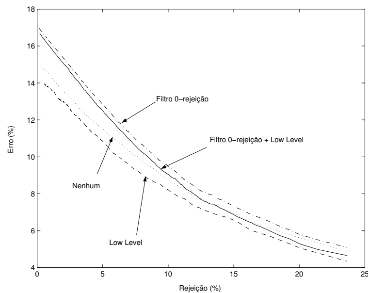
Figura 29: Taxas de reconhecimento de cadeias de caracteres sem o uso de filtro, com o uso de filtro (sem mecanismo de custo), com o uso do low-level verifier e com o uso do filtro+ low-level verifier .
