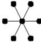
Figura 4.2 Vizinhança 6
