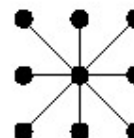
Figura 4.3 Vizinhança 8
