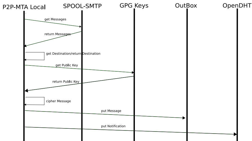
Figura 5.3: Processo para envio de um e-mail
