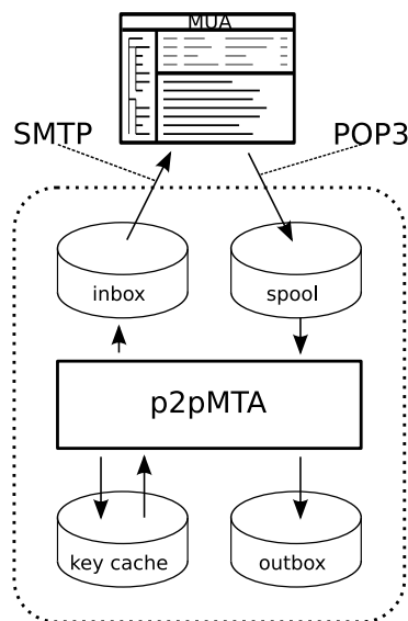
Figura 5.2: Componentes de um p2pMTA
