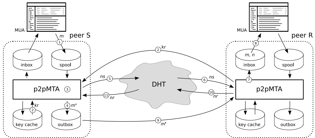
Figura 5.5: Envio e Recebimento de um e-mail
