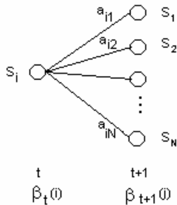
Fig. 3.21 Seqüência de operações requeridas para processamento da variável backward \beta_{t(i)} . Adaptado de [RABINER & JUANG, 1993].
