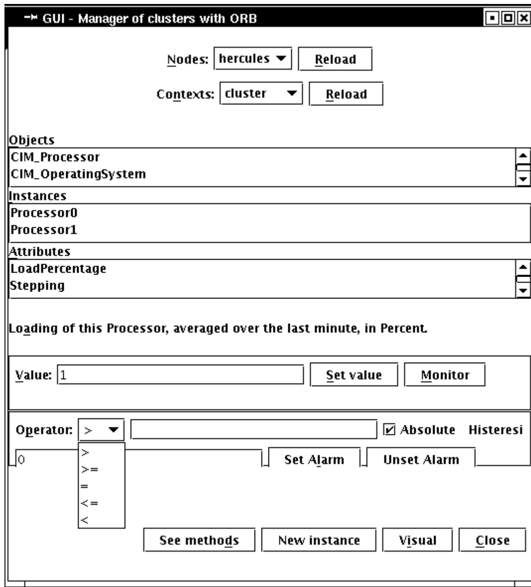
Figura 5.6: Tela principal da GUI
