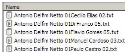
Figura 5.4: Exemplo das combinações para vetores de não-autoria - Testes
