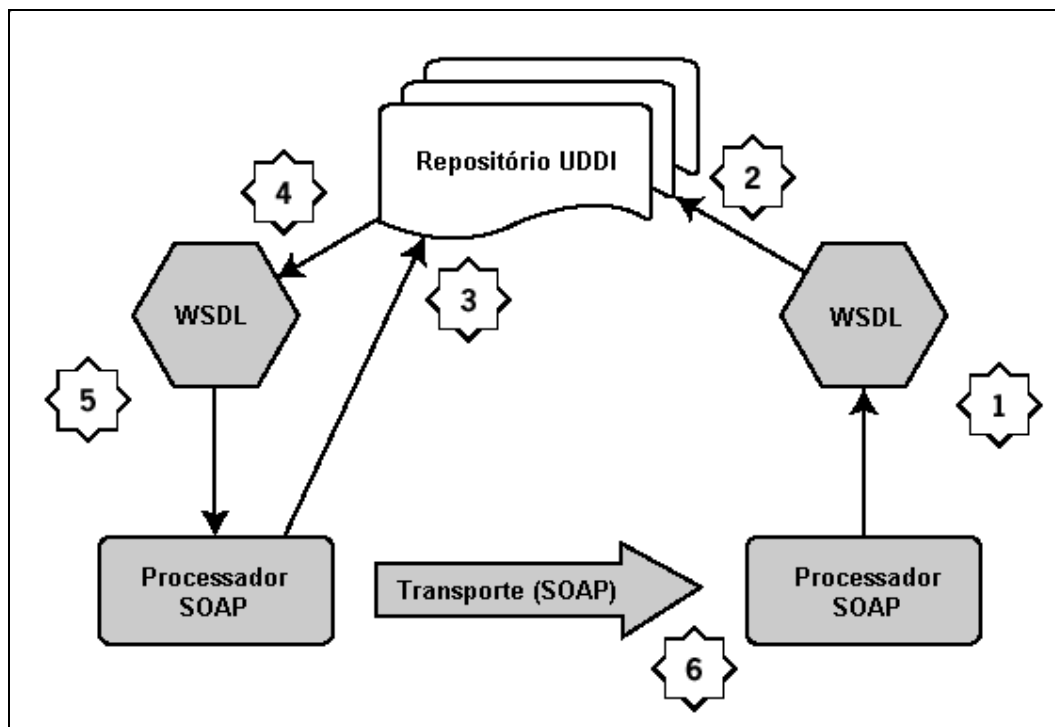
Figura 4.3 – Publicando, localizando e interagindo com web services [NEW02]
