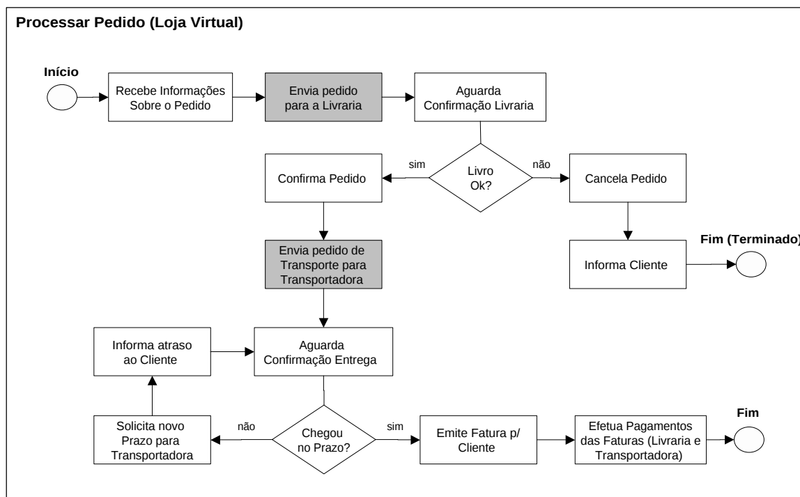
Figura 6.3 – Descrição do processo executado na Loja Virtual para compra de um livro
