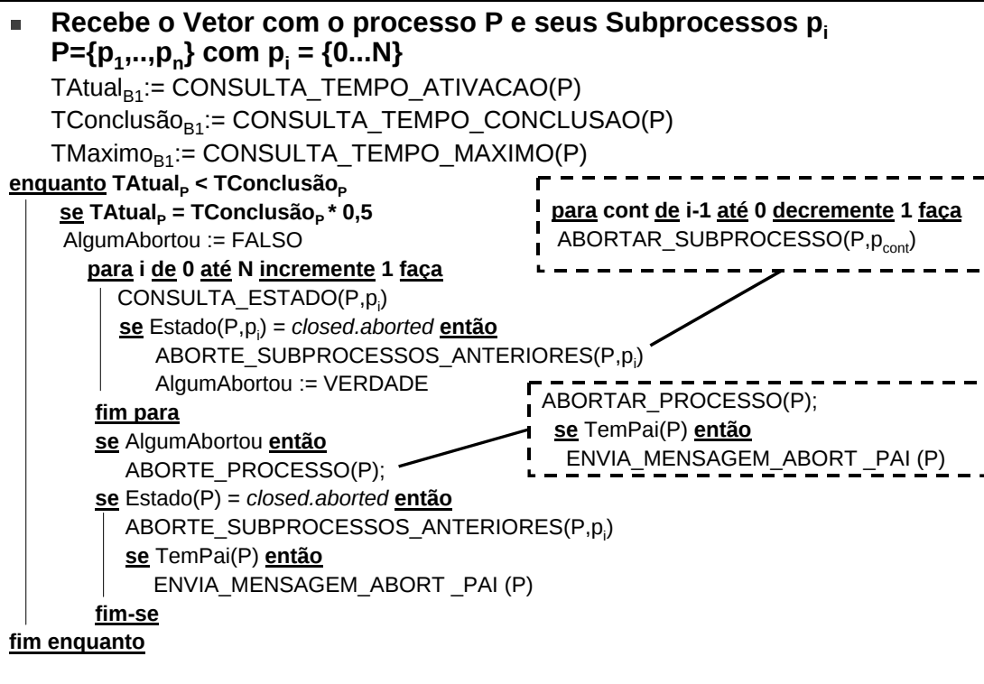
Figura 5.13 – Algoritmo Executor (Tempo Atual < Tempo Conclusão)
