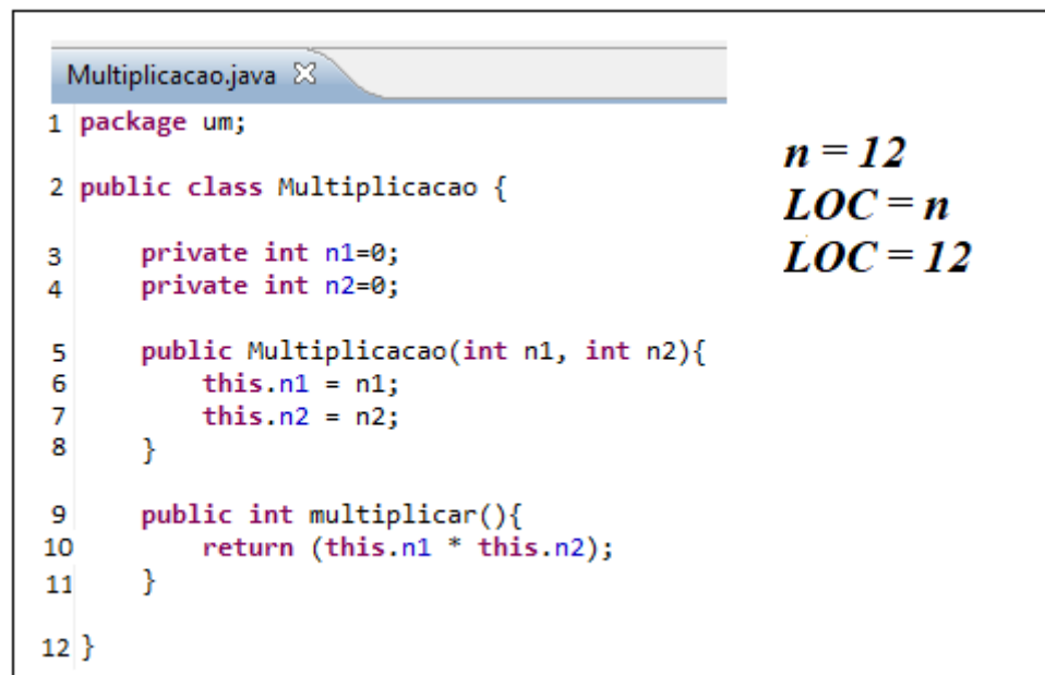
Figura 2.11: Cálculo de LOC para a classe Multiplicacao.java
