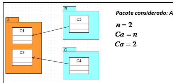
Figura 2.18: Exemplo de Acoplamento Aferente
