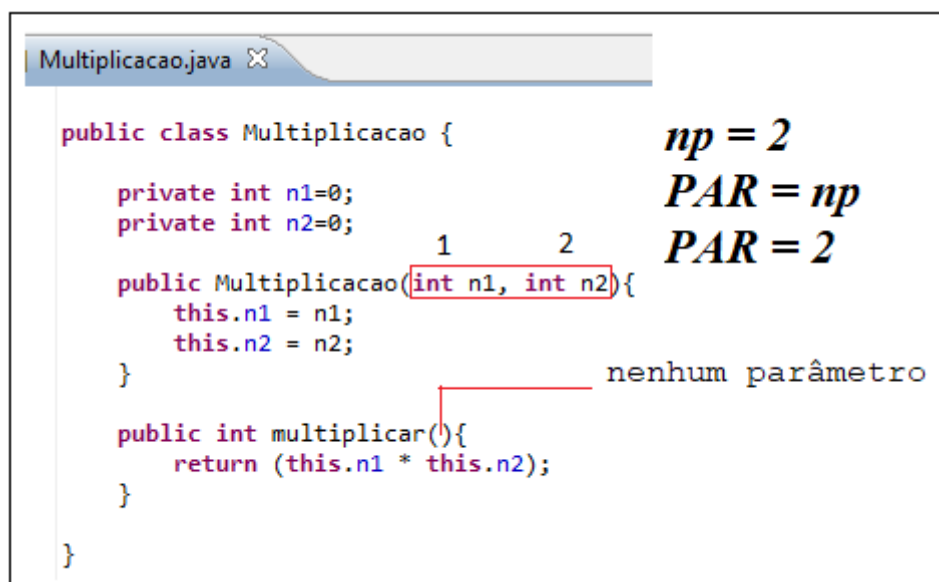
Figura 2.16: Classe Multiplicacao.java com PAR = 2
