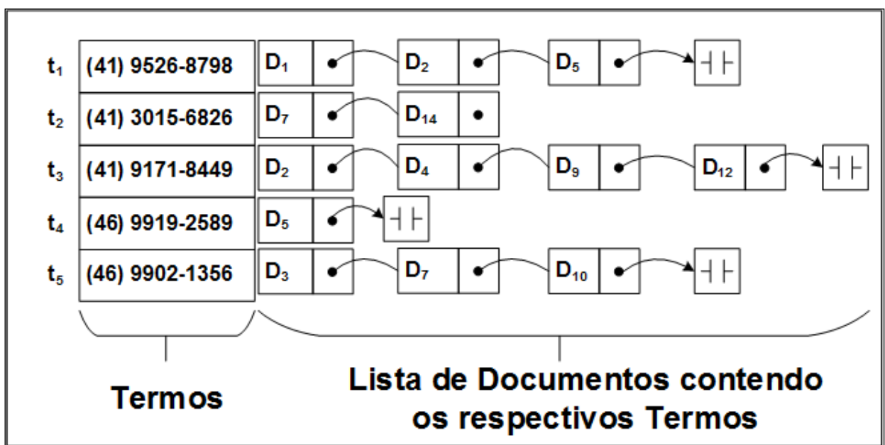
Figura 4.7: SiCReT - Índice Invertido.
