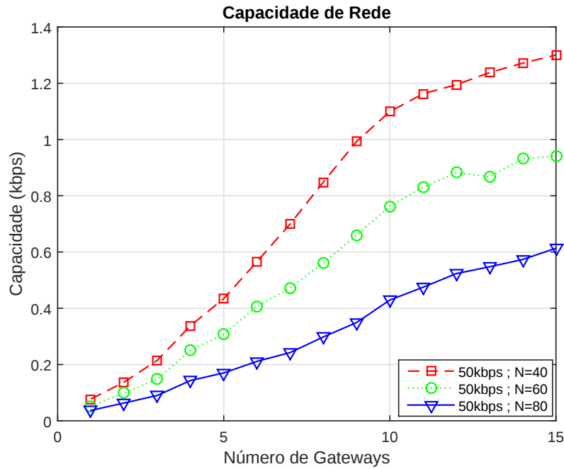
Figura 3.25: Capacidade de Rede (Cenário 1).
