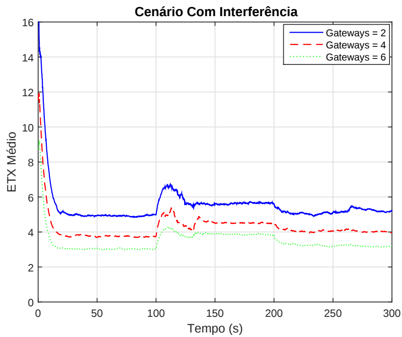
Figura 4.5: ETX médio dos caminhos de roteamento.
