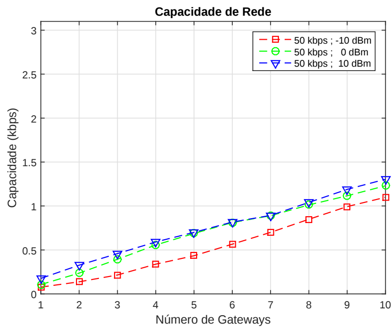
Figura 3.22: Capacidade de rede: Cenário 1.
