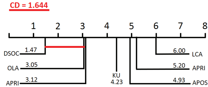
Figura 5.10: Representação gráfica do teste de Nemenyi comparando o desempenho de todos os métodos adotando-se os pools gerados pelo AG proposto. Os valores apresentados próximos dos nomes dos métodos correspondem ao seu ranking médio considerando os 30 problemas de classificação.
