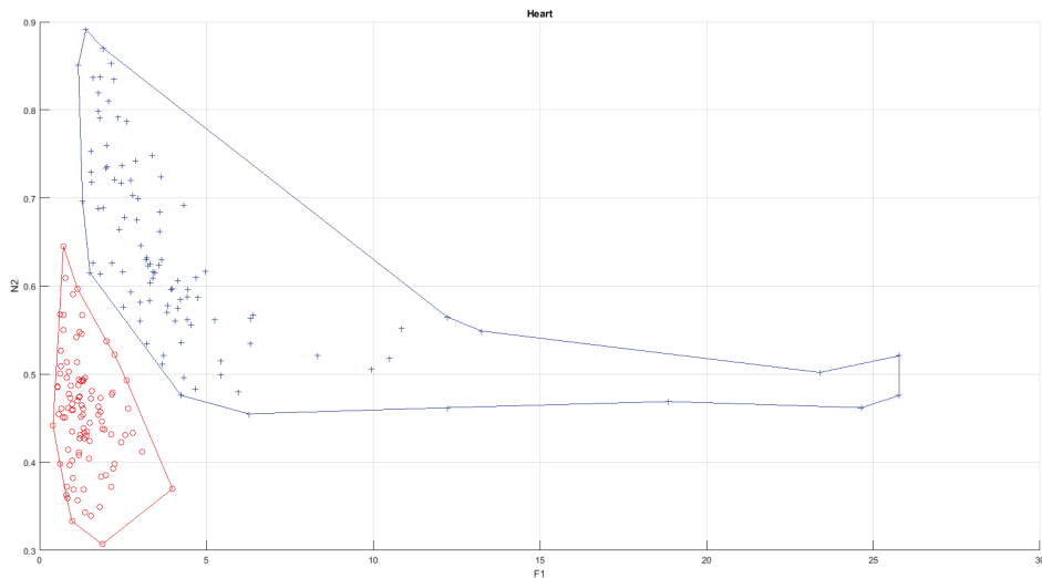
Figura 5.3: Dispersão dos classificadores gerados para a base Heart no espaço de complexidade. Em vermelho os elementos gerados de forma randômica e, em azul, o pool obtido pelo AG.
