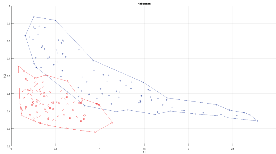
Figura 5.2: Dispersão dos classificadores gerados para a base Haberman no espaço de complexidade. Em vermelho os elementos gerados de forma randômica e, em azul, o pool obtido pelo AG.
