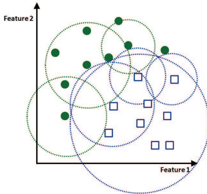
Figura 3.7: Representação da aderência por esferas para duas classes
