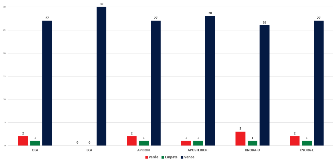
Figura 5.8: Comparação par-a-par da estratégia de SMC proposto perante todos os métodos de seleção testados, baseados na formação randômica do pool . As barras em azul representam os número de problemas em que a adoção da complexidade na geração e seleção superou o método comparado, enquanto as barras em vermelho referem-se ao número de derrotas da abordagem proposta. Os empates são representados pelas barras na cor verde.
