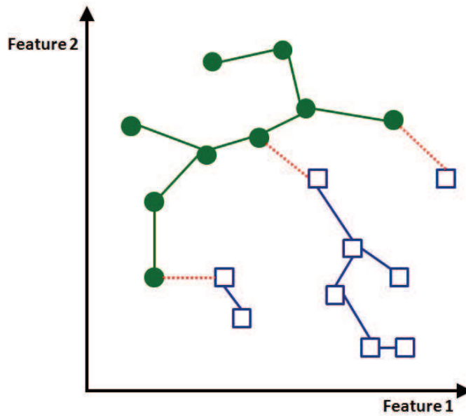
Figura 3.5: Árvore de cobertura mínima construída com base em duas classes
