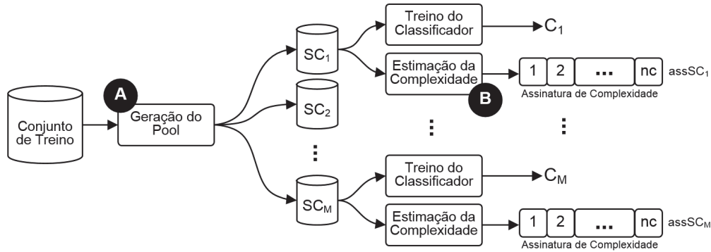
Figura 4.5: Detalhamento de parte da etapa de treinamento - Fluxo de informações que serão adotadas na etapa operacional
