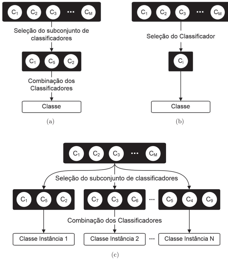
Figura 2.5: Três abordagens para seleção e combinação de classificadores (Adaptado de [(KO; SABOURIN; BRITTO JR., 2008)]): a) seleção estática de conjunto de classificadores; b) seleção dinâmica de classificador único e c) seleção dinâmica de conjunto de classificadores
