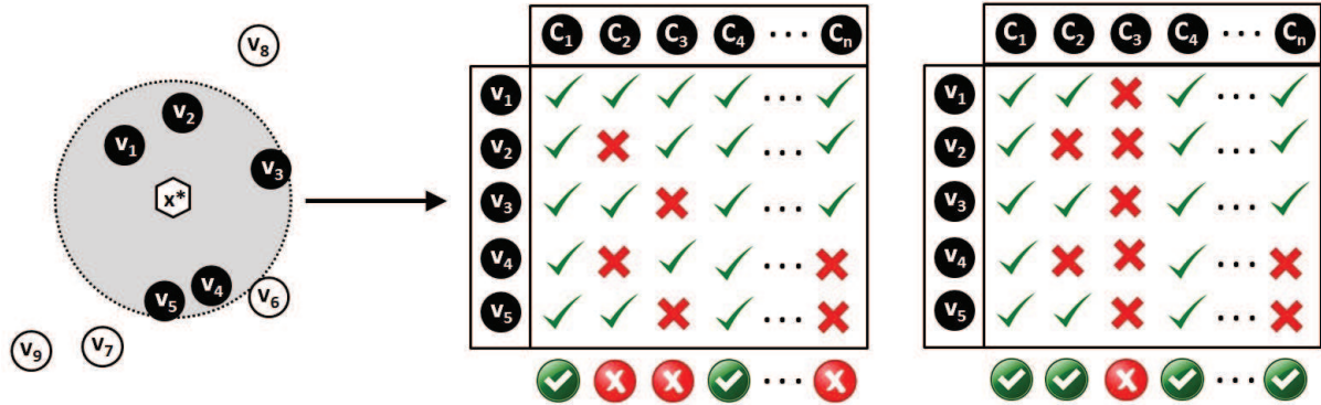
Figura 2.7: Ideia do funcionamento dos métodos KNORA-Eliminate e KNORA-Union
