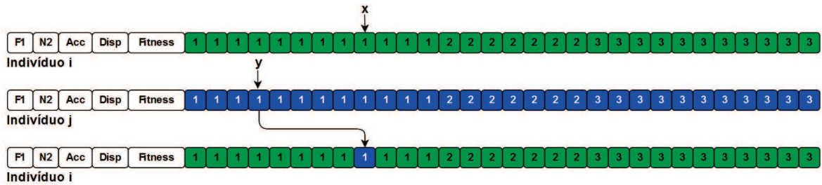
Figura 4.4: Processo de Mutação: a instância selecionada é trocada por outra aleatoriamente escolhida em um indivíduo diferente, necessariamente pertencente à mesma classe.
