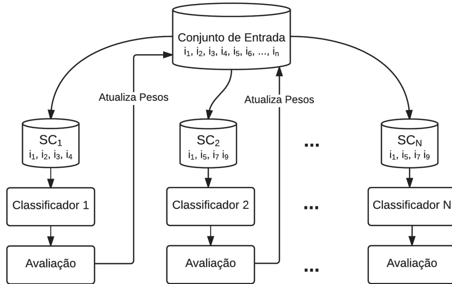
Figura 2.3: Ideia do funcionamento do Boosting
