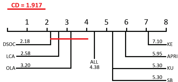
Figura 5.6: Representação gráfica do teste de Nemenyi comparando todos os métodos. Os valores apresentados próximos dos nomes dos métodos correspondem ao seu rank médio considerando os 30 problemas de classificação.
