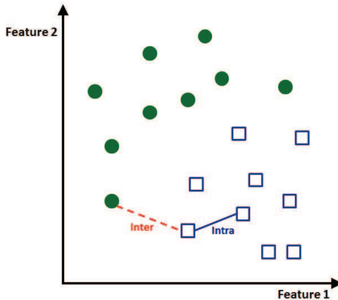
Figura 3.6: Representação da distância entre os vizinhos mais próximos intra e inter-classes
