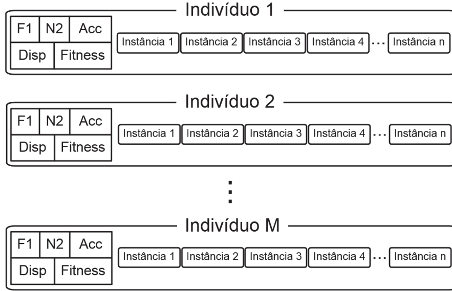
Figura 4.2: Estrutura adotada para o AG.
