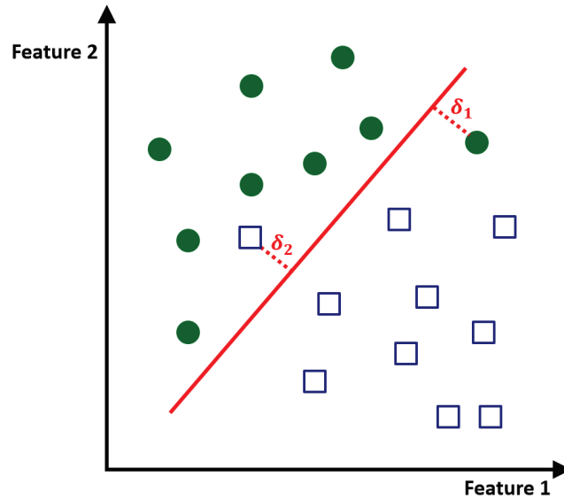
Figura 3.4: Classificador linear ótimo que erra ao classificar as duas instâncias em destaque
