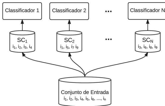
Figura 2.2: Estrutura do funcionamento do Bagging
