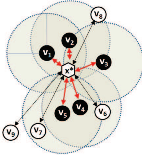
Figura 2.6: Avaliação da vizinhança da instância a ser classificada
