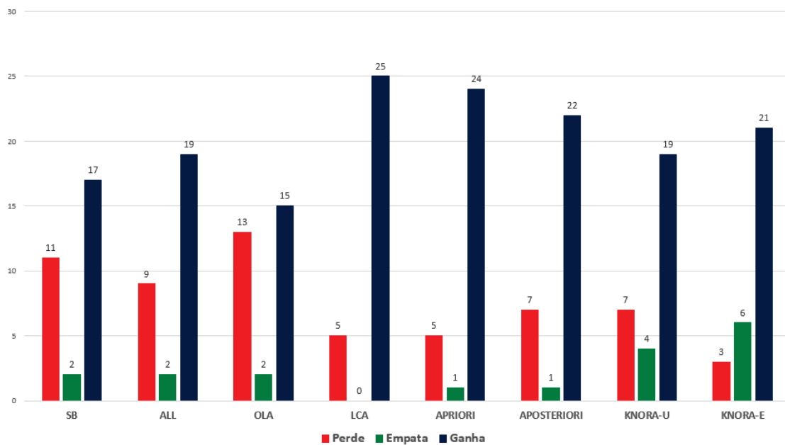
Figura 5.1: Comparação par-a-par da performance dos métodos seleção dinâmica, single best e combinação com base nos dois métodos de geração.
