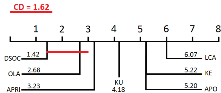
Figura 5.9: Representação gráfica do teste de Nemenyi comparando todos os métodos. Os valores apresentados próximos dos nomes dos métodos correspondem ao seu ranking médio considerando os 30 problemas de classificação.
