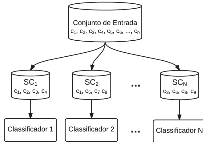
Figura 2.4: Construção de classificadores via Random Subspaces
