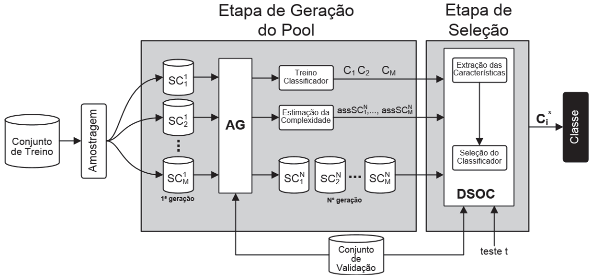
Figura 4.1: Estrutura macro do método desenvolvido, apresentando os processos de geração, seleção e classificação.
