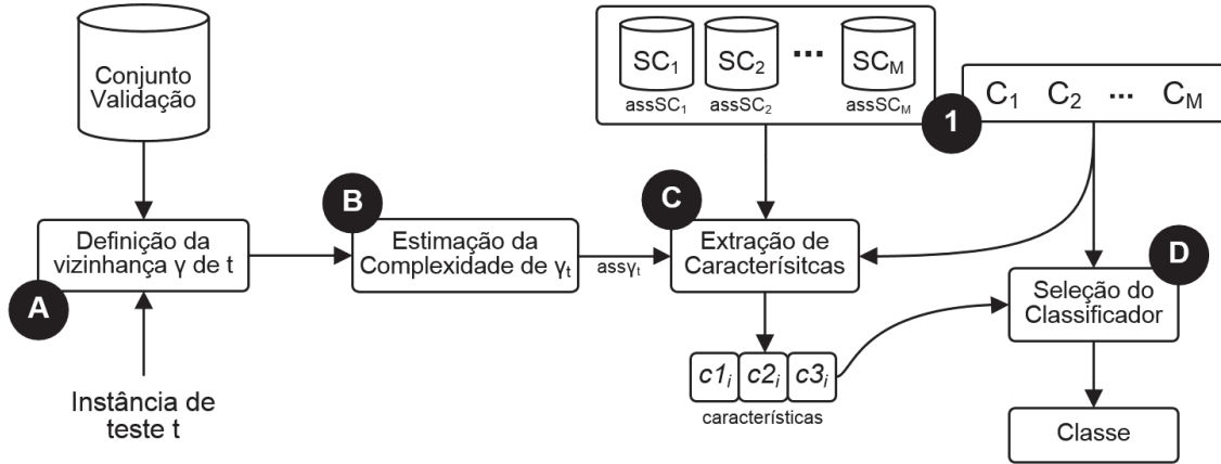
Figura 4.6: Ilustração da etapa operacional do SMC - levantamento das características e estimação da competência dos classificadores
