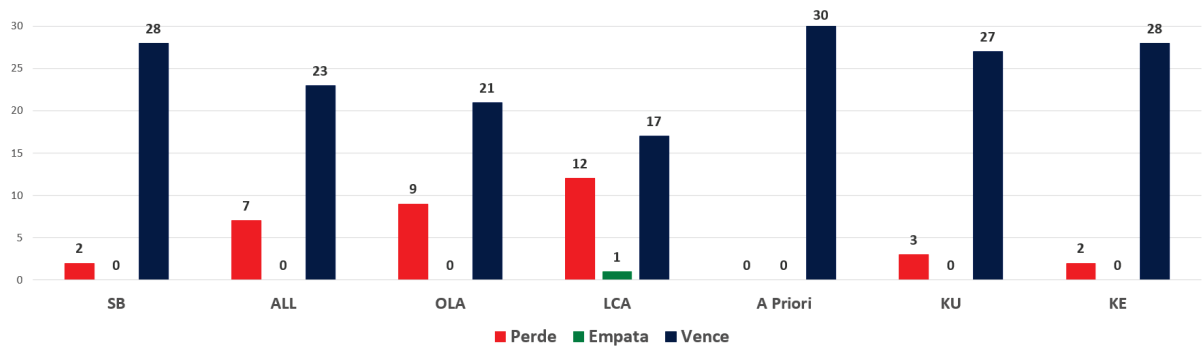
Figura 5.5: Comparação par-a-par do DSOC com todos os métodos testados. As barras em azul representam os número de problemas em que a adoção da complexidade na seleção superou o método comparado, enquanto as barras em vermelho referem-se ao número de derrotas da abordagem proposta. Os empates foram representados pelas barras na cor verde.
