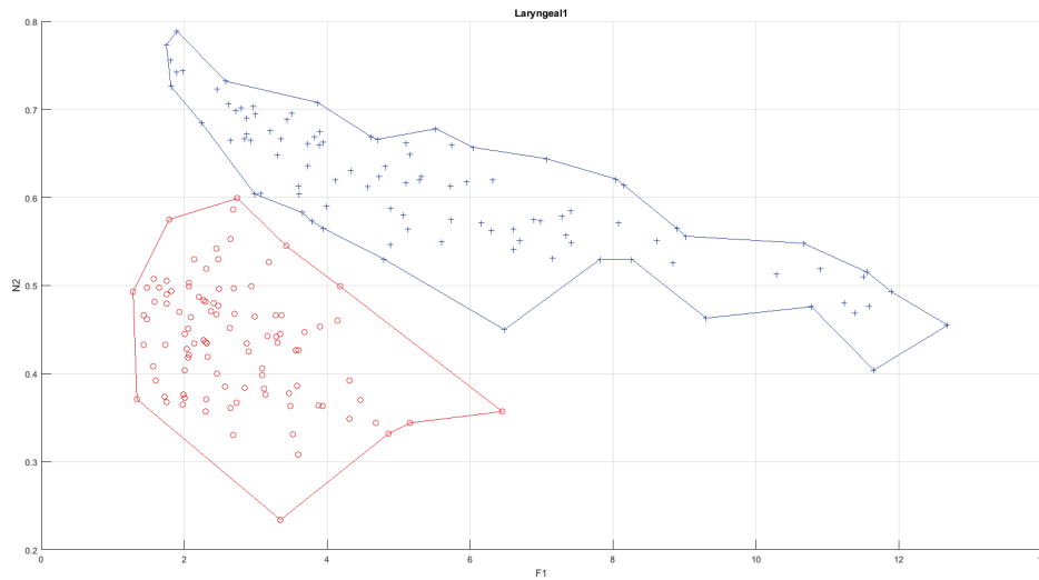
Figura 5.4: Dispersão dos classificadores gerados para a base Laryngeal1 no espaço de complexidade. Em vermelho os elementos gerados de forma randômica e, em azul, o pool obtido pelo AG.
