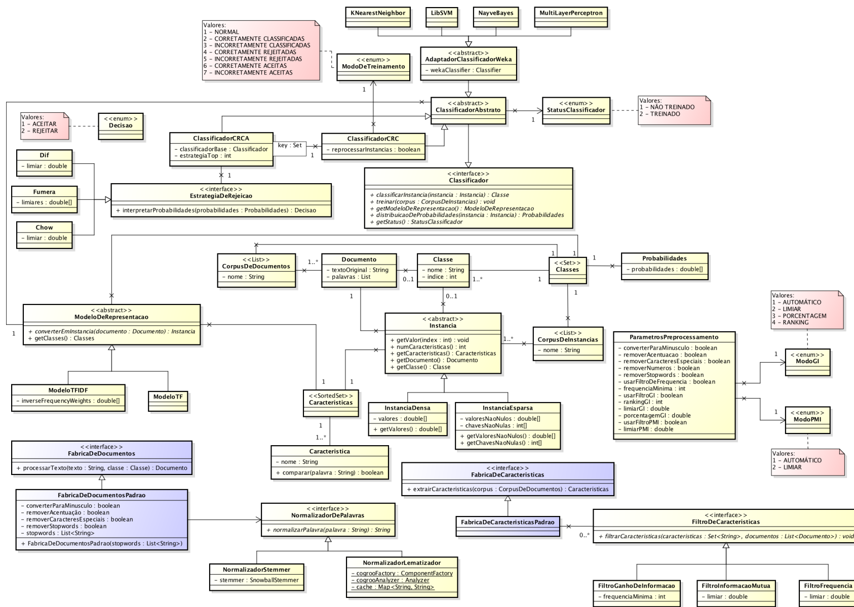
Figura 6.4: Diagrama de classes do método de identificação de emoções em textos
